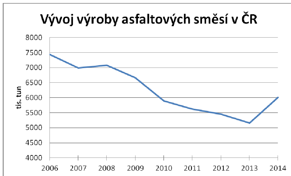
Graf 7 Vývoj výroby asfaltových směsí v ČR v letech 2006 až 2014 [81]
