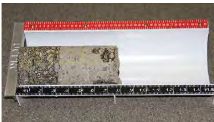
Obrázek 22 Přípravek pro orientační měření jádrových vývrtů a jejich fotodokumentaci [49]
