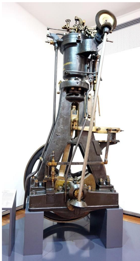
Obrázek 2 - Druhý prototyp Dieselova motoru [27]
