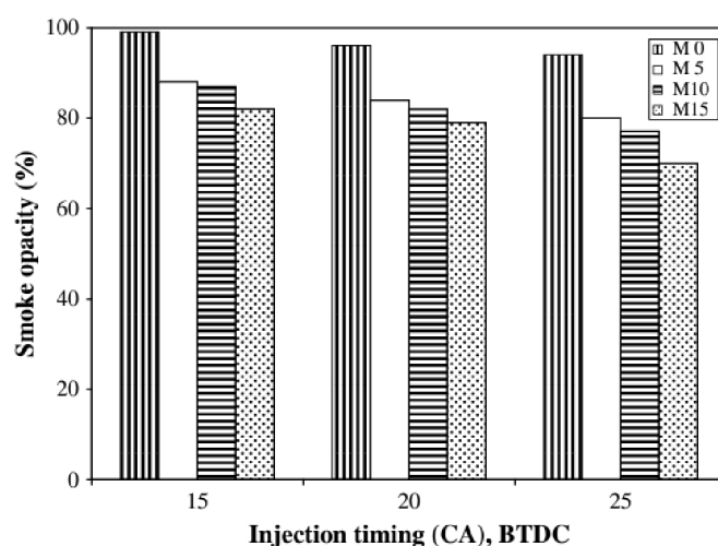
Obrázek 23 - graf závislosti úhlu předstihu vstříku paliva na kouřivosti motoru při zátěži 20 Nm [20]
