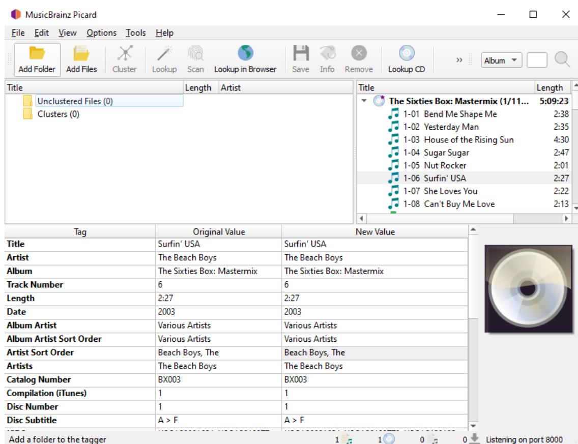
Obrázek 3.2: MusicBrainz Picard, multiplatformní software na tagování hudebních souborů. Podporuje dohledání metadat v databázi MusicBrainz. Také podporuje AcousticID, což je nástroj na vytváření a vyhledávání otisků (audio fingerprint) hudebních souborů.
