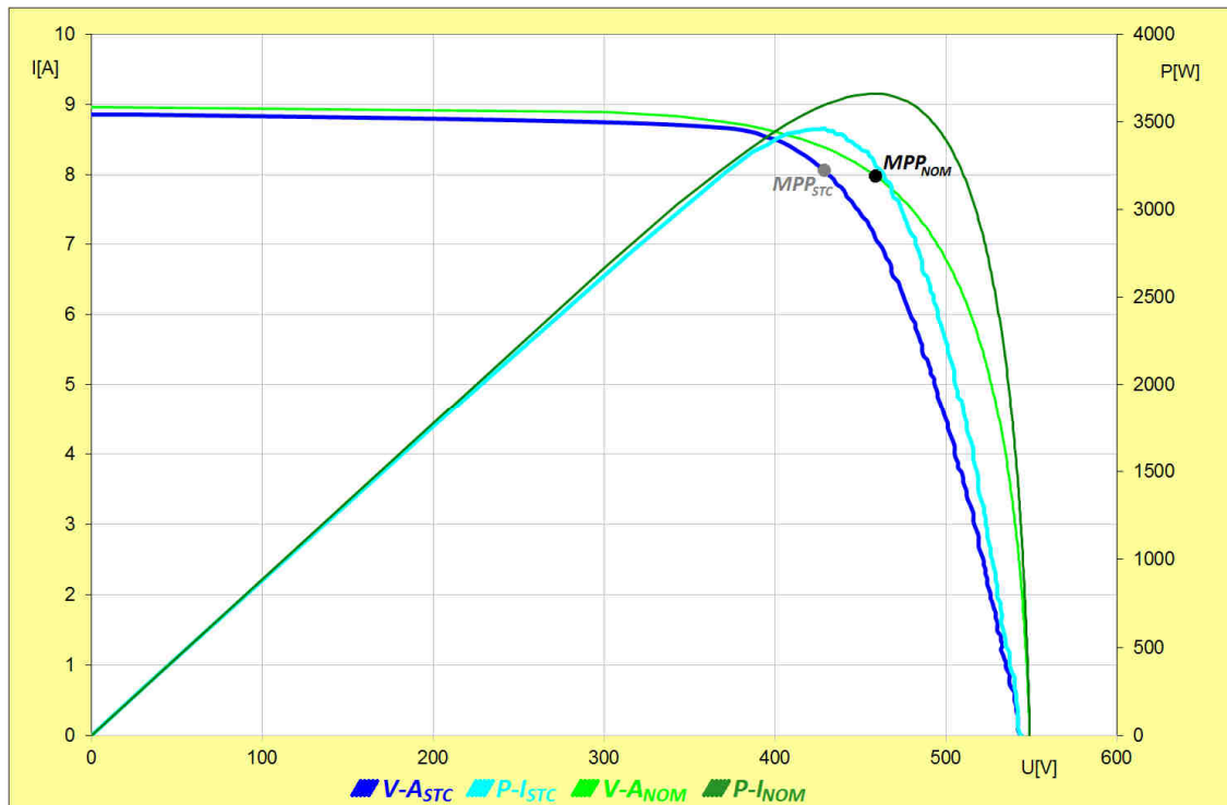
Obr. 5.2-4 V-A charakteristika FV stringu č.3
