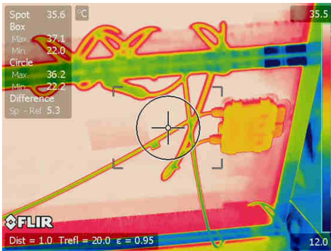
Obr. 5.2-8 Snímek připojovacího boxu a konektorů FV modulu 2.8
