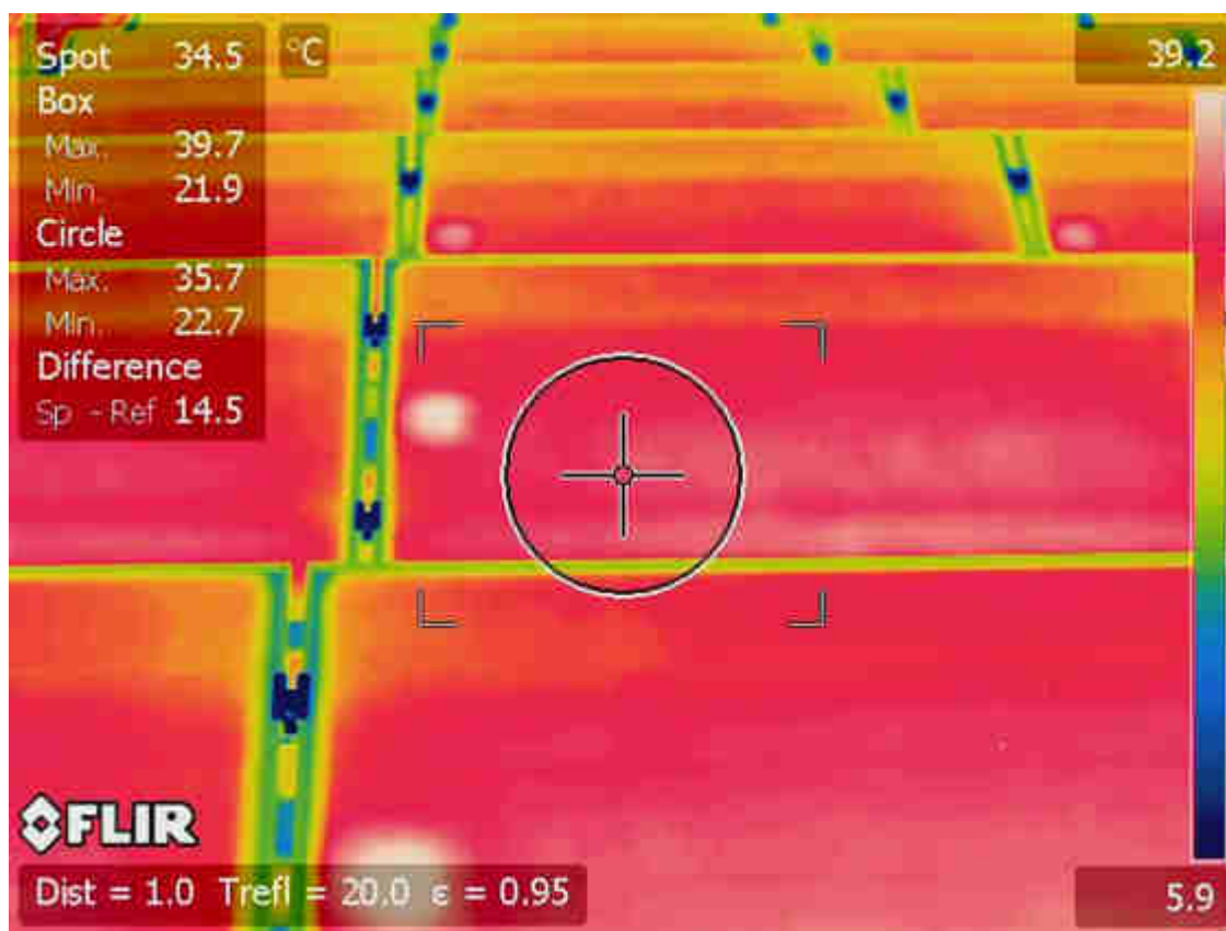
Obr. 5.2-9 Termovizní pohled na část FV pole
