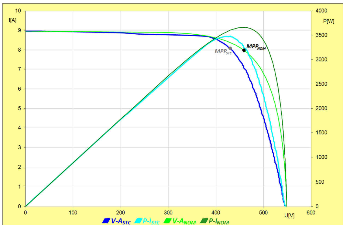
Obr. 5.2-3 V-A charakteristika FV stringu č.2
