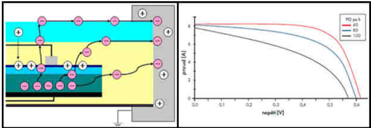
Obr. 2.2-1 Potenciální indukovaná degradace [20][22][19]
