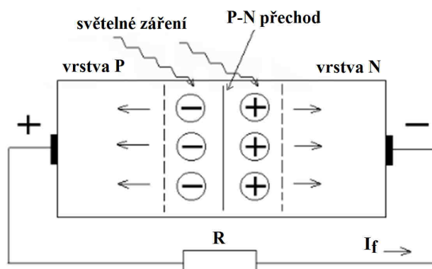
Obr. 1.1-1 Fotovoltaický jev [33]
