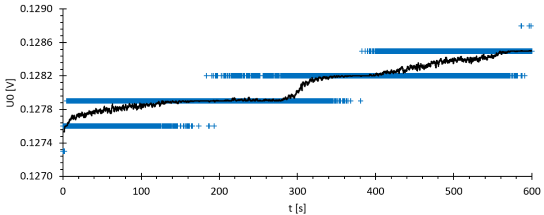
Obr. 4.2: Napětí na referenčním můstku, vzorkovací frekvence 52 Hz, průtok 80 kg/h. Modré body jsou měřené napětí, černá čára představuje průběžné průměrování pro 64 vzorků.
