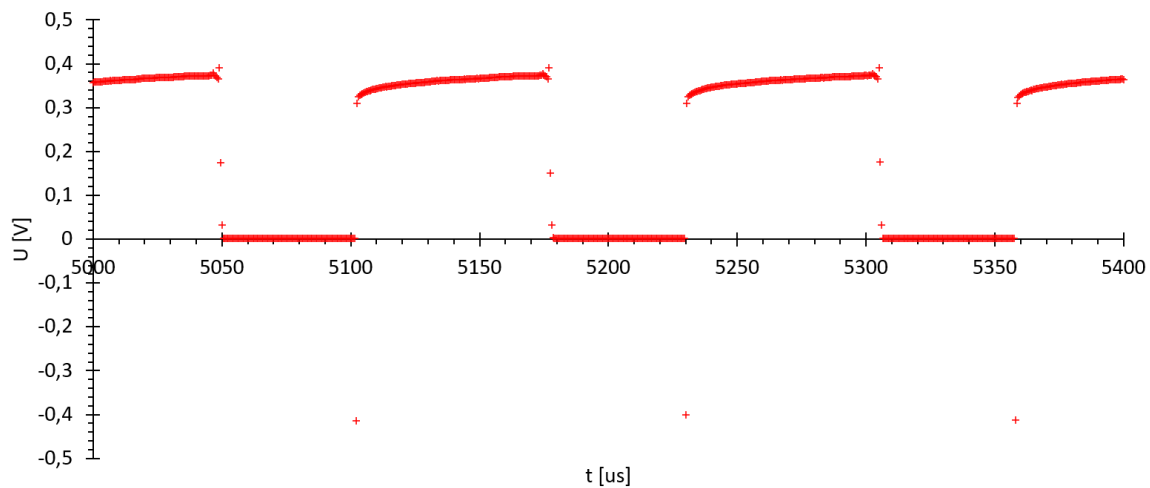
Obr. 4.4: Napětí na vyhřívaném můstku.
