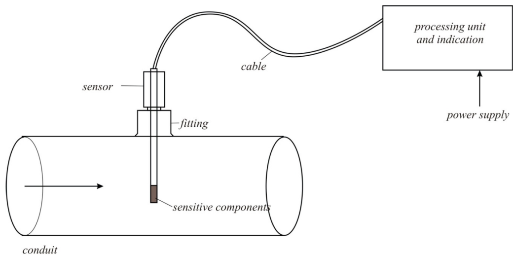
Obr. 1.2: Ukázka termoanemometrického principu.[3]
