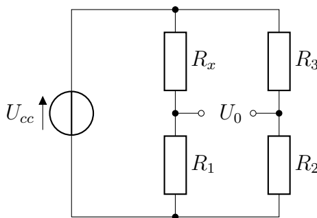
Obr. 2.1: Schéma Wheatstonova můstku, R_x je neznámý odpor, R_1 , R_2 a R_3 jsou známé odpory. U_0 je rozdílové napětí můstku, U_{cc} je napájecí napětí můstku.
