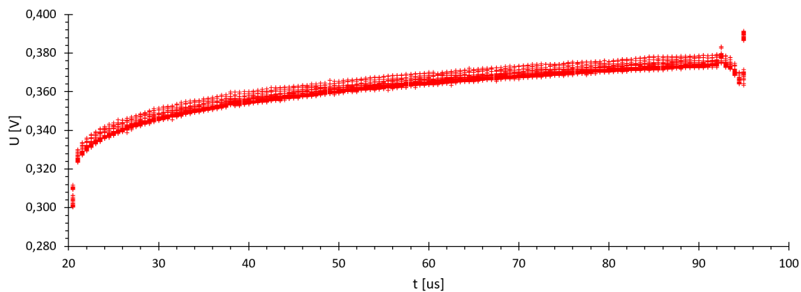
Obr. 4.5: Napětí na vyhřívaném můstku, složený průběh.
