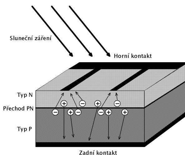
Obr.1.1 Struktura solárního článku
