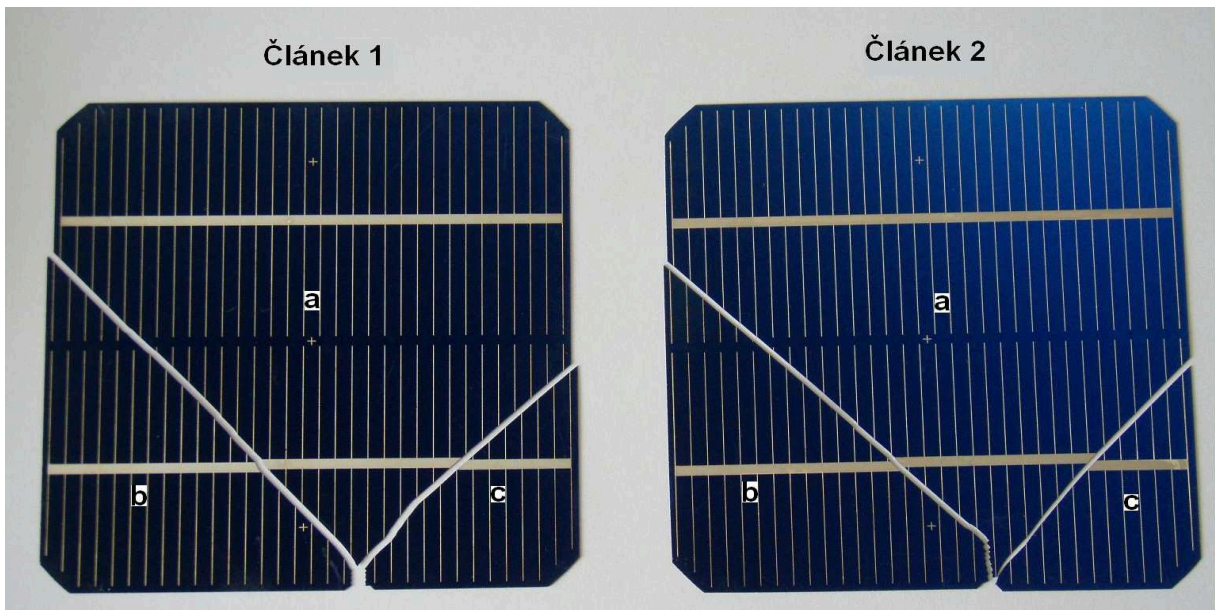
Obr.7.4 Testovací články
