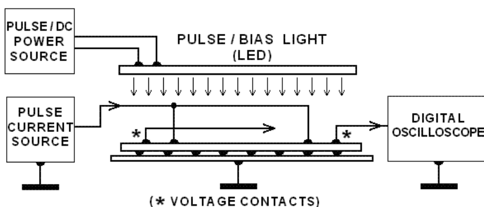
Obr.2.3 Blokové schéma měřicího zařízení (převzato z [3])
