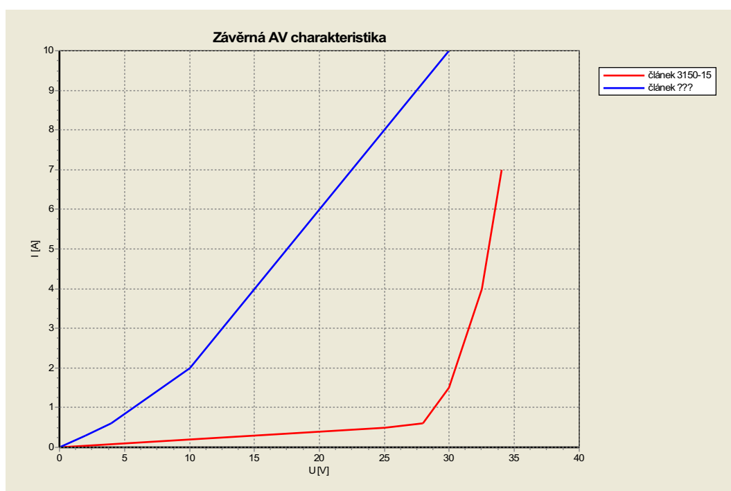
Obr.6.2 Závěrné napětí – AV charakteristiky
