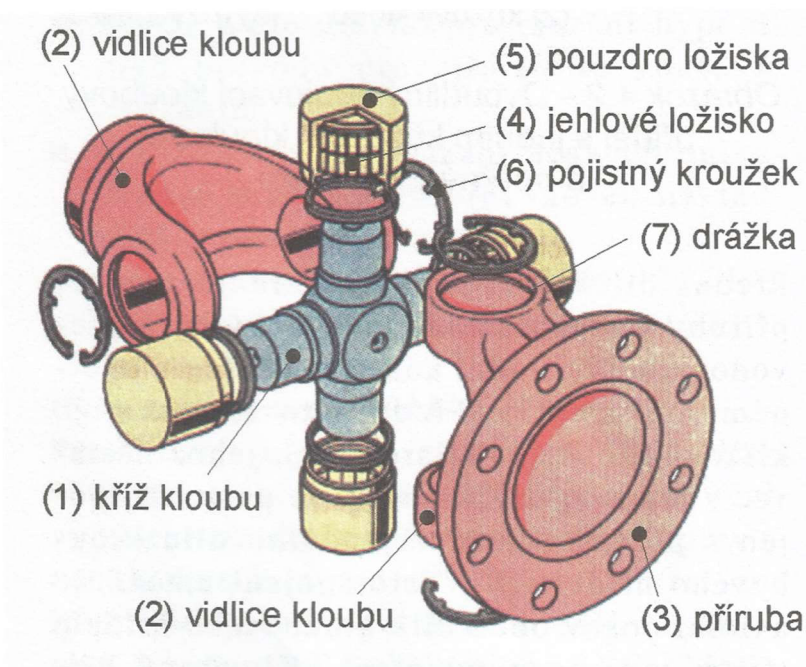
Obr. 5 Rozbiratelný křížový kloub [1]
