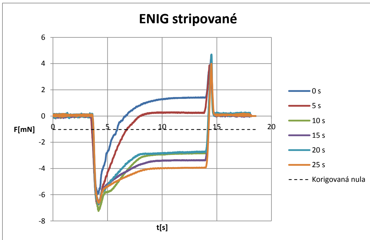
Obr 7.15 Smáčecí charakteristiky stripovaných vzorků ENIGu v závislosti na čase v lázni
