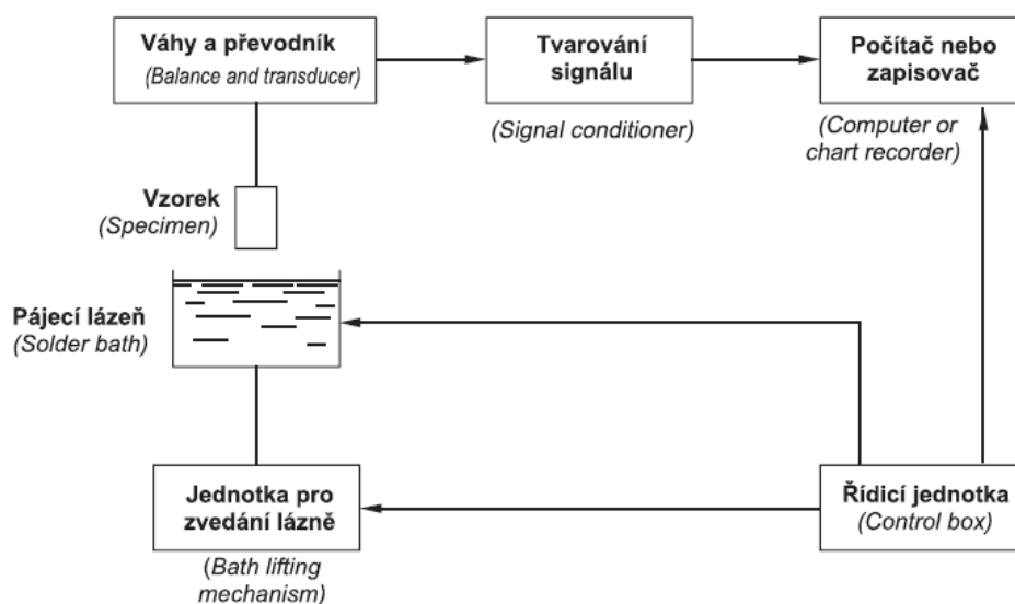
Obr 6.1 Schéma meniskografu [4]
