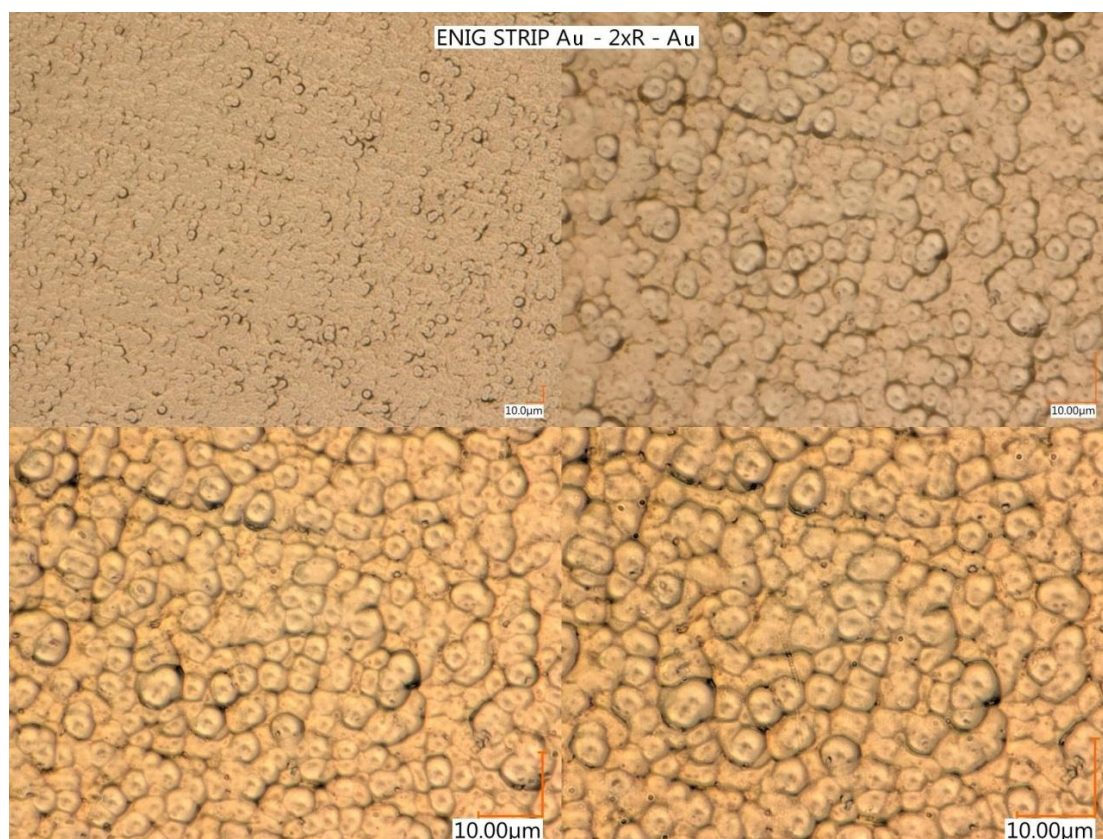
Obr 7.20 Povrch ENIGU u kterého se nepodařilo odstripovat vrstvu zlata (reflow 2x)
