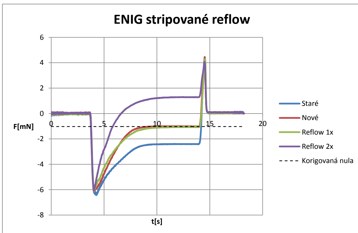
Obr 7.16 Smáčecí charakteristiky stripovaného ENIGu po průchodech přetavovací pecí
