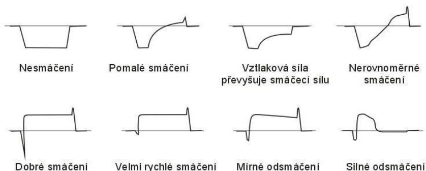
Obr 6.3 Různé průběhy smáčení [3]
