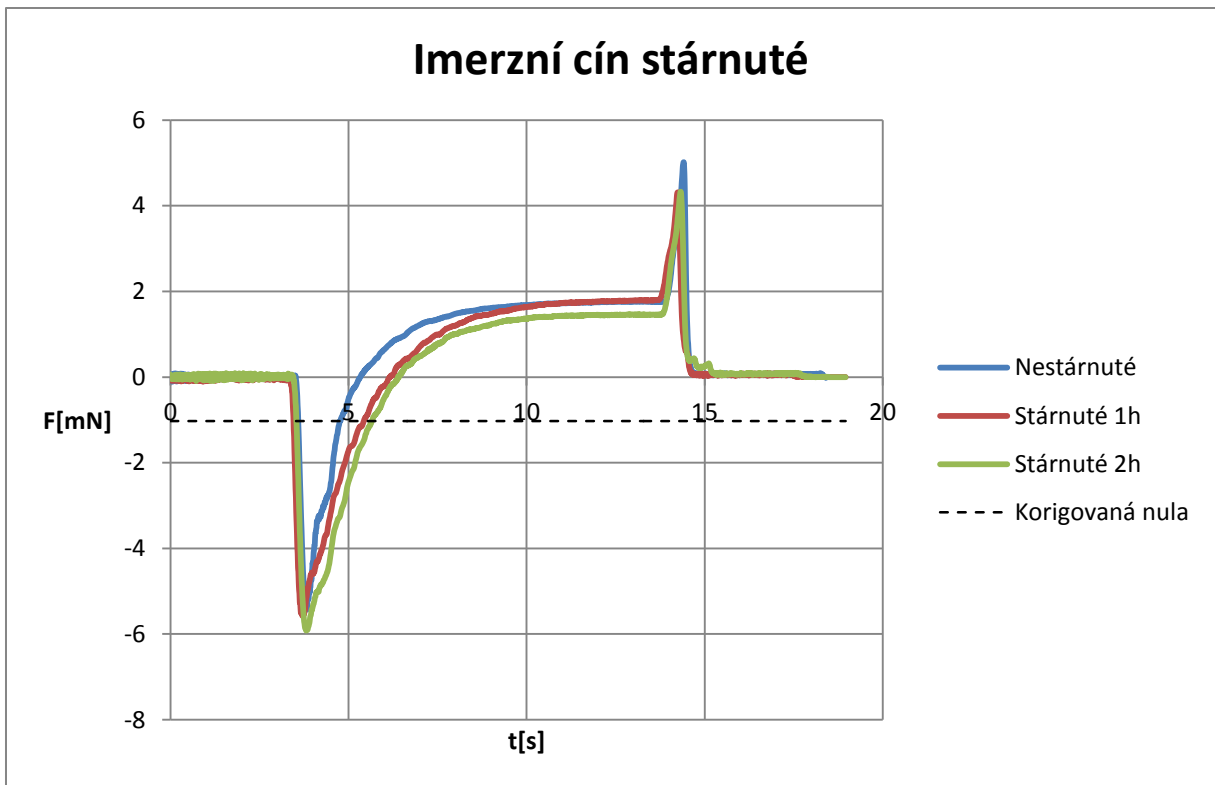
Obr 7.11 Smáčecí charakteristiky imerzního cínu po izotermálních stárnutí
