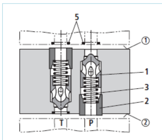
Obrázek 18 Zpětný ventil [12]
