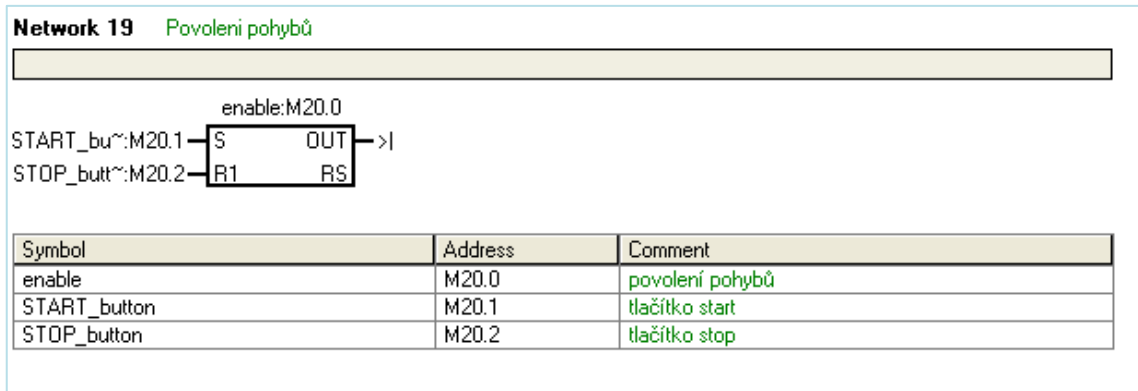
Obrázek 46 Povolení pohybů
