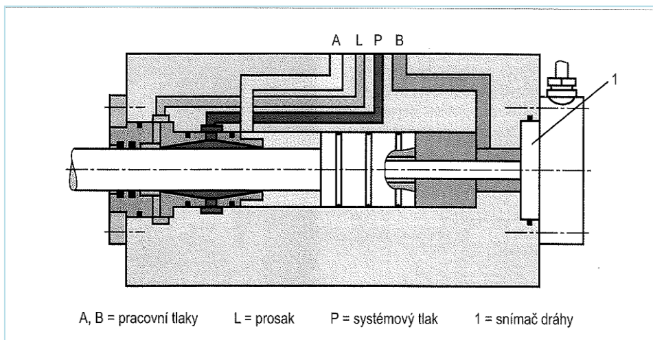
Obrázek 19 Servoválec s hydrostatickým vedením pístnice – kuželový prostor [4]
