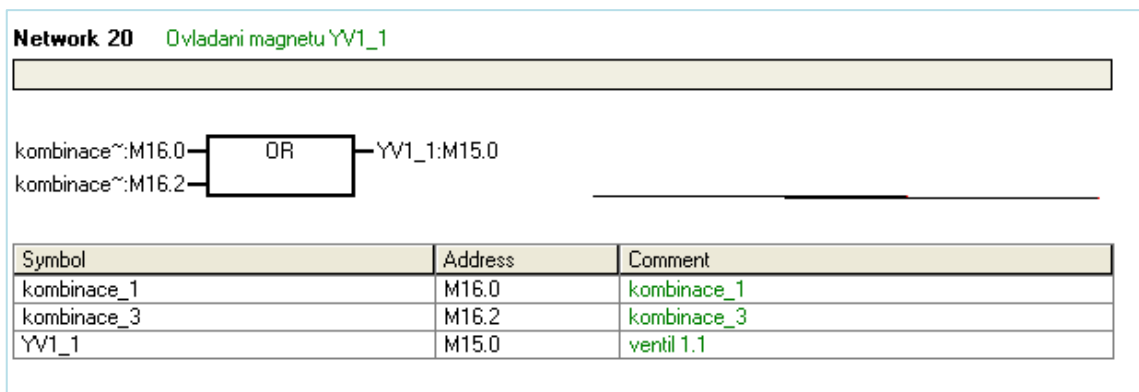
Obrázek 45 Ovládání magnetu
