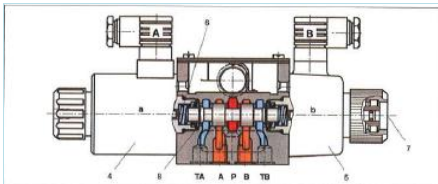
Obrázek 11 Šoupátkový rozvaděč – 3 komorový [4]
