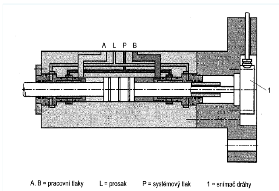
Obrázek 20 Servoválec s hydrostatickým vedením pístnice – válcový prostor [4]
