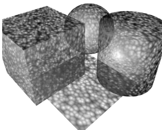
Obr. 2.4: Transparentná textúra
