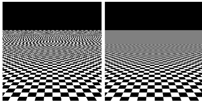
Obr. 2.15: Využitie mipmappingu
