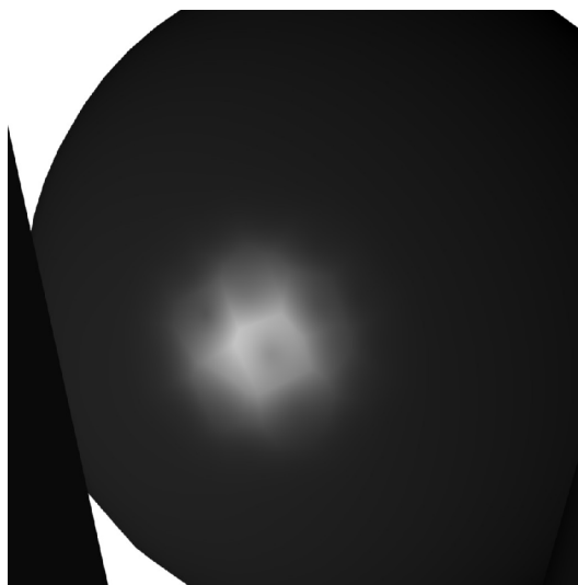
Obr. 2.3: Spekulárna textúra
