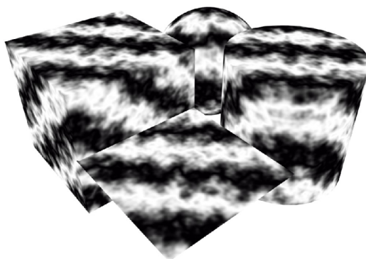
Obr. 2.2: Ambientná textúra
