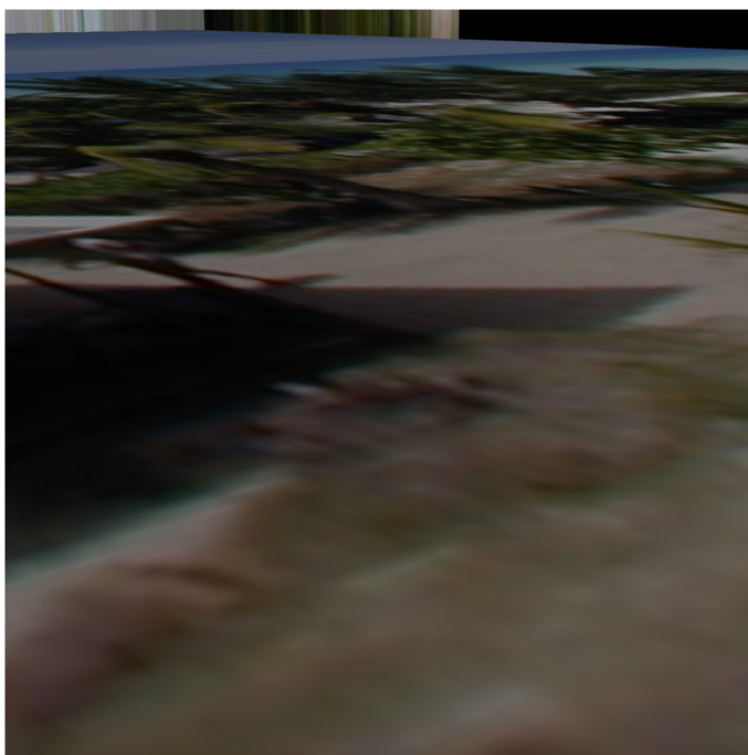
Obr. 2.13: Bilineárne filtrovanie
