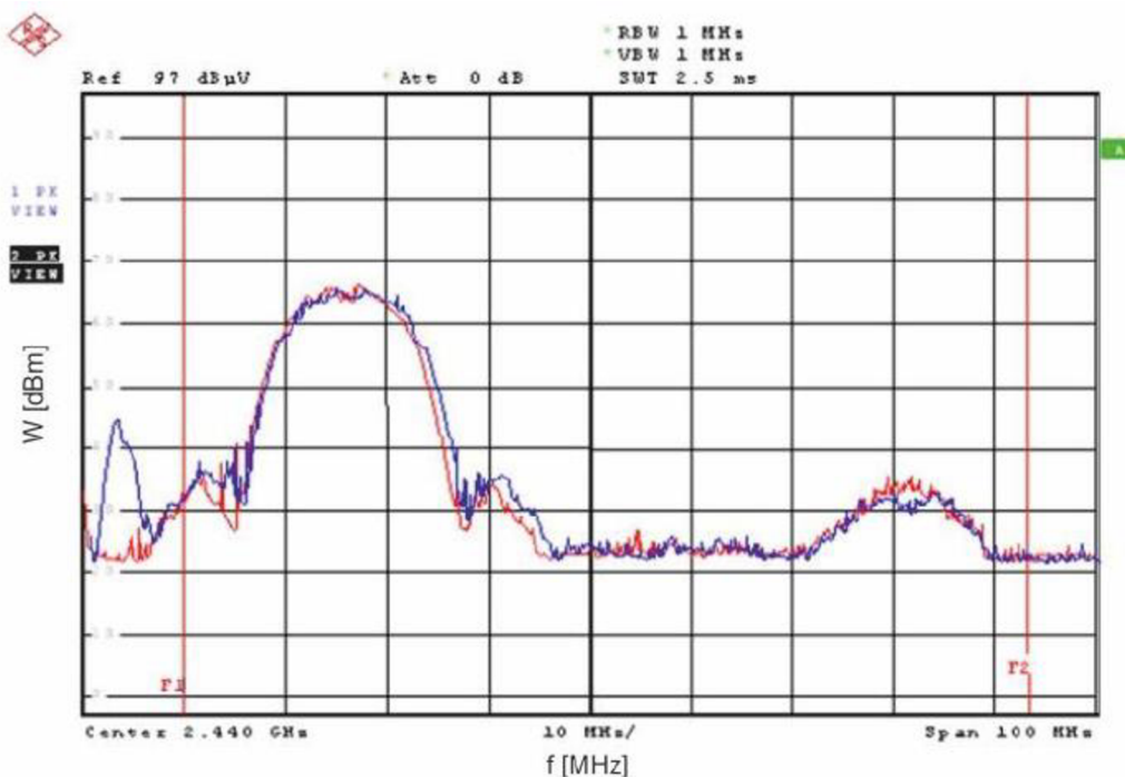
Obr. 2.7: Spektrum signálů na MB1 – polarizace vertikální / polarizace horizontální.
