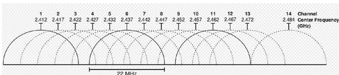
Obr. 2.5: Grafické znázornění rozdělení kanálů podle DSSS.
