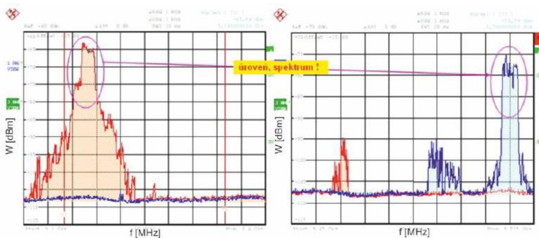
Pozn. Červeně je znázorněno spektrum kmitočtu před přeladěním, modře po přeladění.
