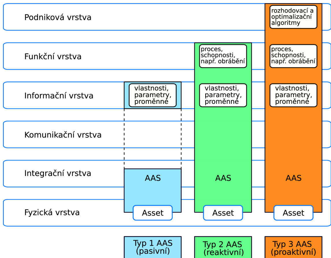
Obr. 1.4: Typy AAS zobrazené ve vrstvé ose RAMI 4.0 (inspirace z literatury [9])
