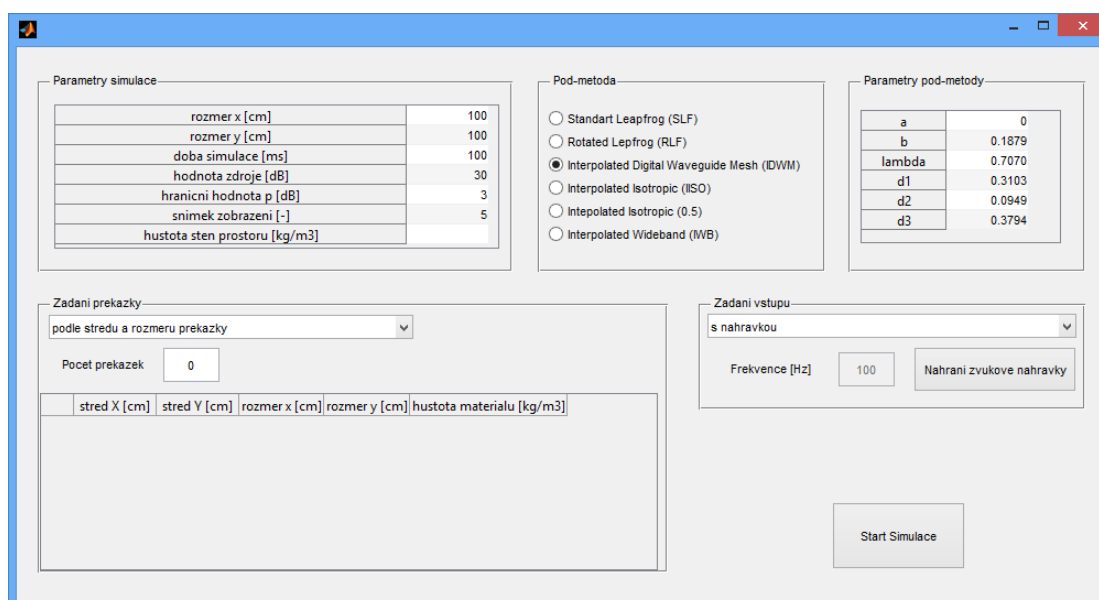
Obr. 4.1: Grafické rozhraní algoritmu metody FDTD
