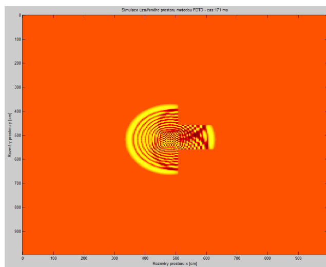
Obr. C.2: Zobrazení simulace jevu difrakce o roh překážky (metoda IDWM) v čase 171 ms
