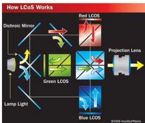
Obr. 12: Schéma LCoS projektoru [30]
