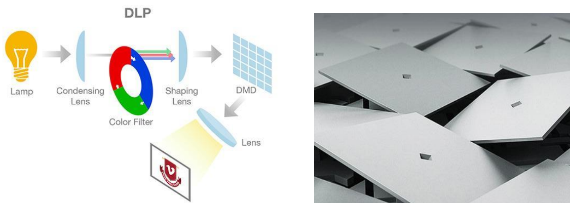
Obr. 11: Vlevo - Schéma DLP projektoru [29], vpravo - DMD pod mikroskopem [26]
