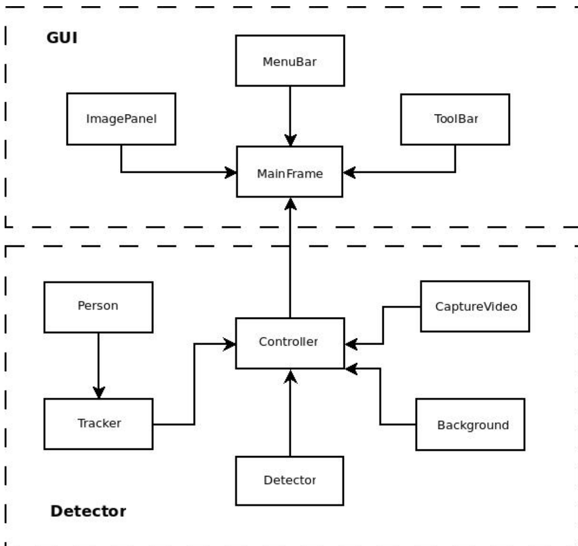
Obrázek 5.1: Diagram komponent
