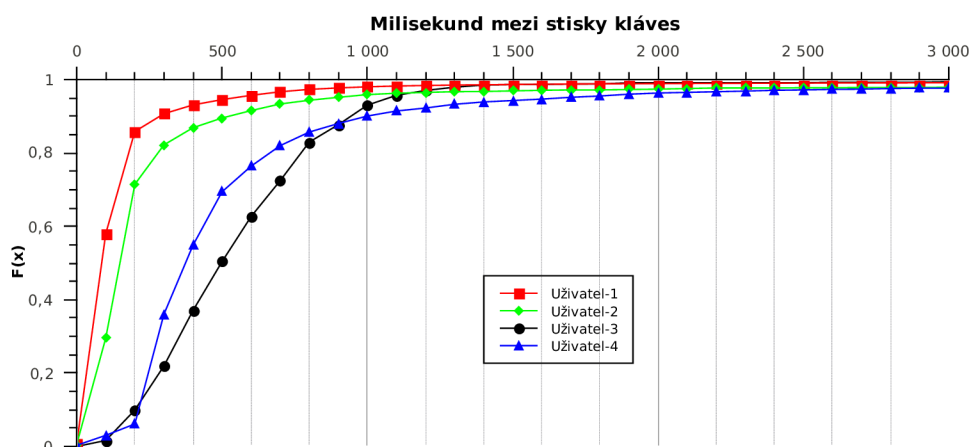
Obrázek 3.1: Graf distribuční funkce popisující čas mezi stisky kláves čtyř různých uživatelů. Čím rychlejší růst křivky v blízkosti osy Y, tím rychlejší a lepší psaní uživatele.
