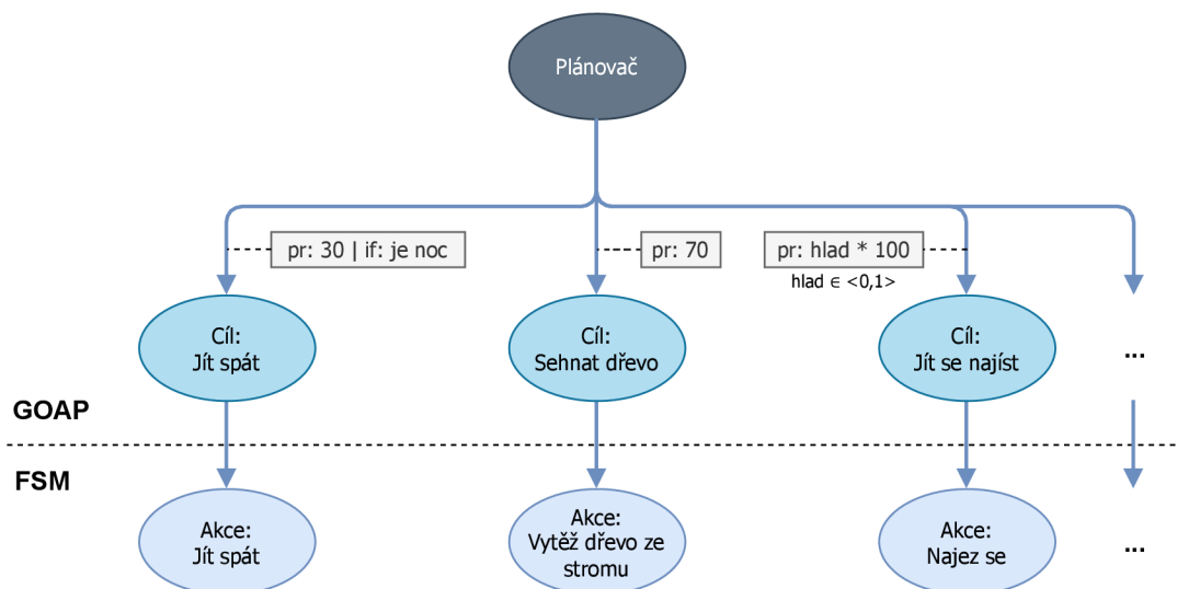
Obrázek 6.3: Schéma řídicího systému autonomních agentů. Přerušovanou čarou je naznačeno rozdělení na GOAP a FSM vrstvy systému. U hran vedoucích od plánovače k cílům jsou vidět priority cílů označené „pr:“ a podmínka jejich aktivace označená „if:“.
