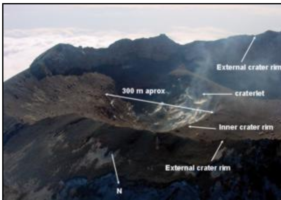
Obr. 6: Kráter Popocatépetlu v počáteční fázi sopečné aktivity (14. ledna 2005).
