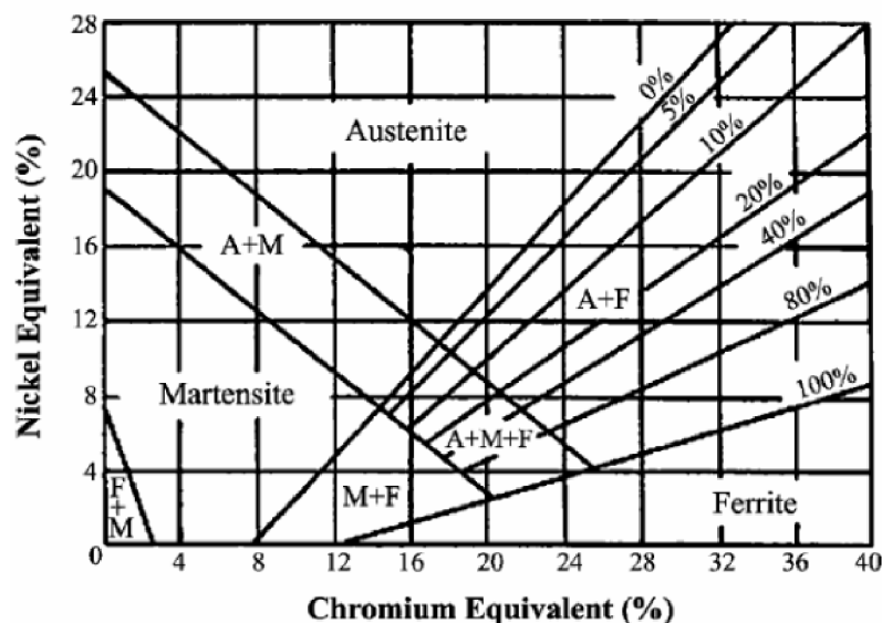
Obr. 5 Schaefflerův-Delongův diagram [3]
