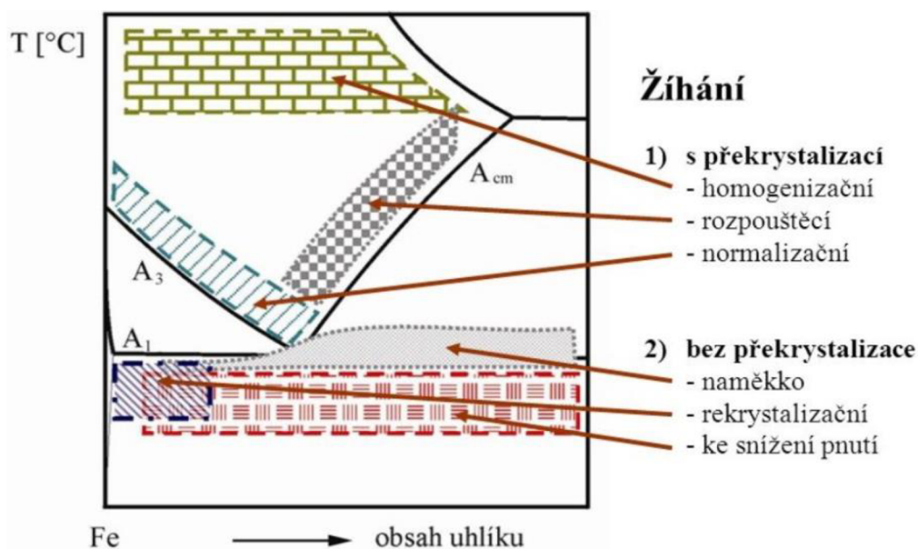
Obr. 18 Základní typy žihání [24]
