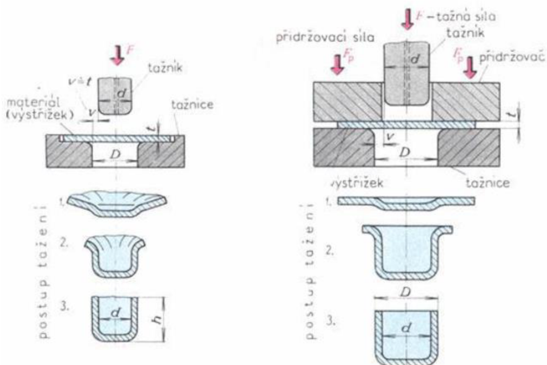
Obr. 22 Tažení bez přídržovače (vlevo) a s přídržovačem (vpravo) [28]
