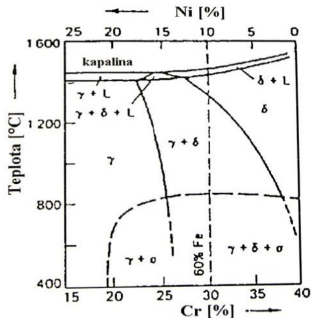
Obr. 2 Řez ternárním diagramem Fe-Cr-Ni [3]
