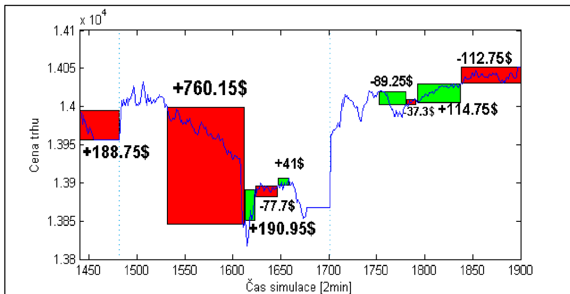
Graf 4.6 - Ukázka obchodů základního predikčního modelu v průběhu dvou dní.
