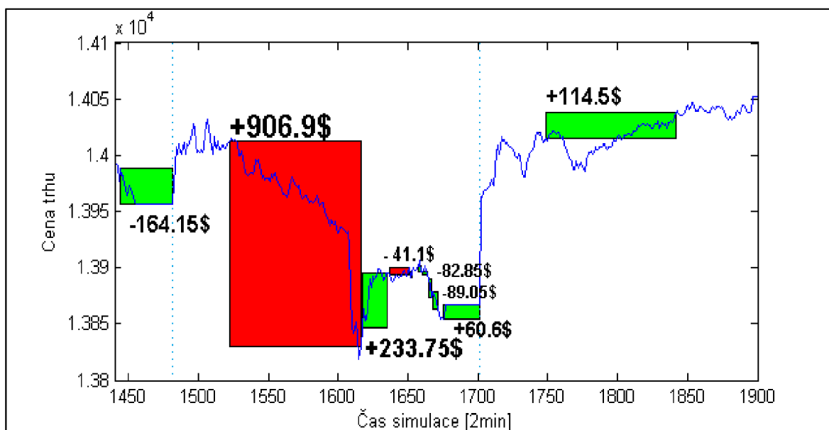
Graf 4.7 - Ukázka obchodů upraveného predikčního modelu v průběhu dvou dní.
