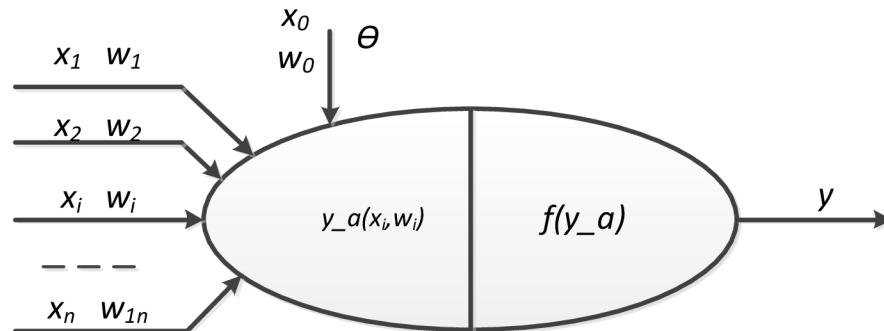
Obrázek 3.2 - Schéma umělého neuronu. Funkce y_a(x_i, w_i) je agregační funkce a f(y_a) je aktivační funkce neuronu. Vstupem jsou vážené hodnoty x a výstupem je hodnota y .
