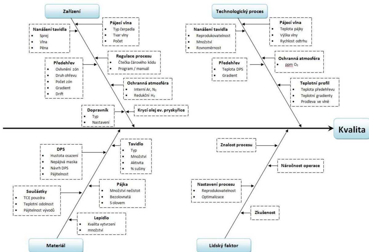
Obr. 3.: Ishikawa diagram pro kontrolu kvality u strojního pájení vlnou
