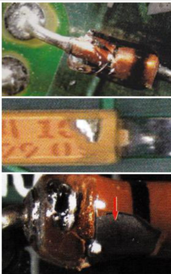
Obr. 49.: Příklady vyštipnutí – nesmí nastat [10]
