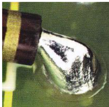
Obr. 23.: Pájka v ohybu vývodu – nesmí nastat [10]
