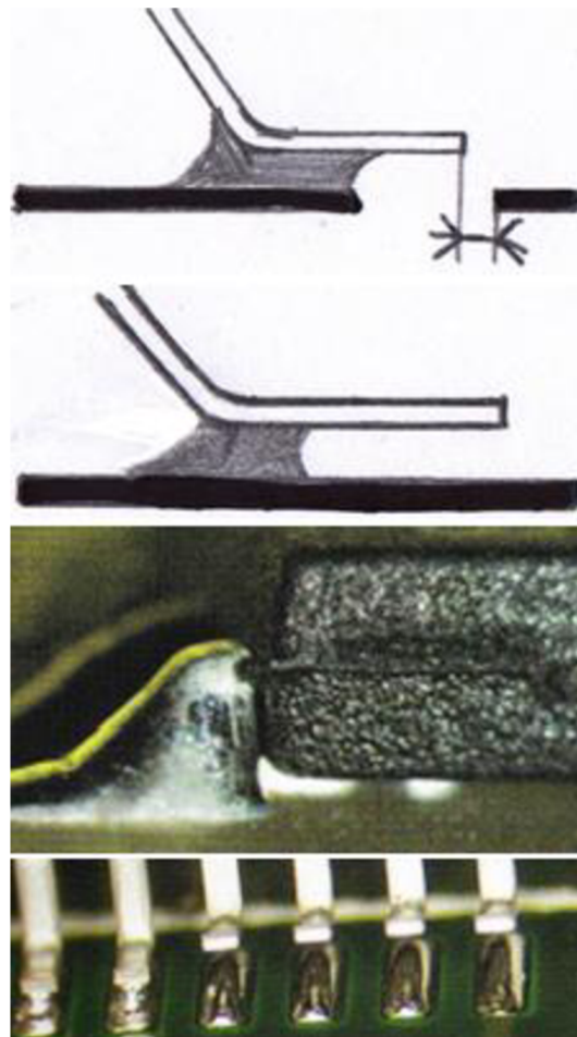
Obr. 30.: Příklady co nesmí nastat
