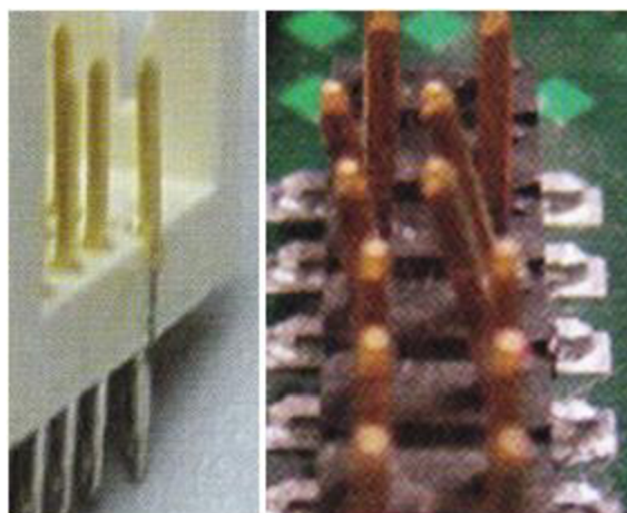
Obr. 50.: Příklad poškození konektoru [10]
