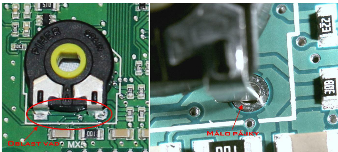
Obr. 54.: Oblast vad na trimru a špatné propájení
