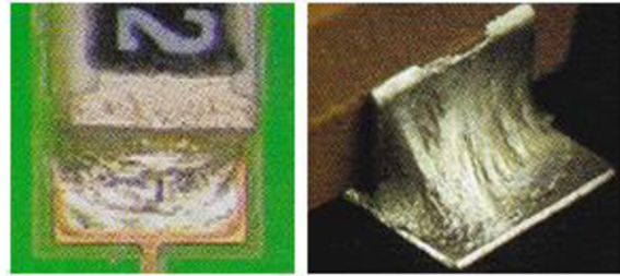
Obr. 20.: Narušené tuhnutí [10]
