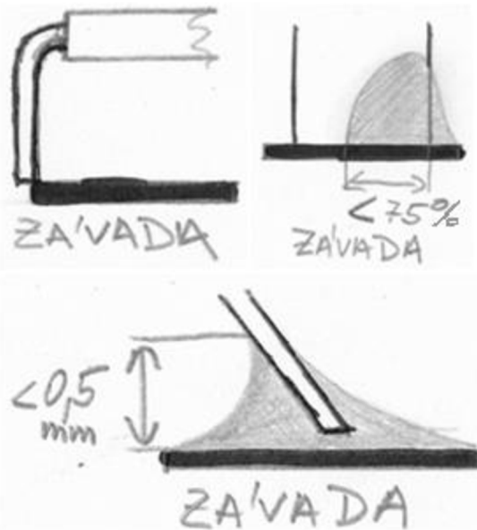
Obr. 29.: Příklady závad u spoje na tupo
