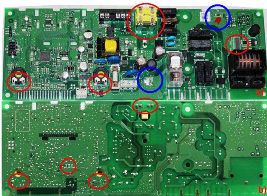
Obr. 51.: Znáornění výskytu častých chyb na DPS: a) primární strana, b) sekundární strana
