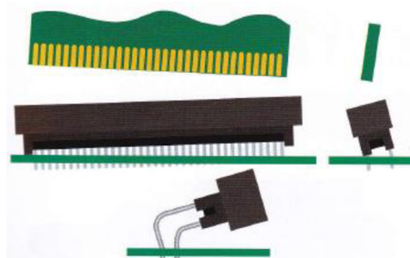
Obr. 36.: Nakloněné konektory [10]
