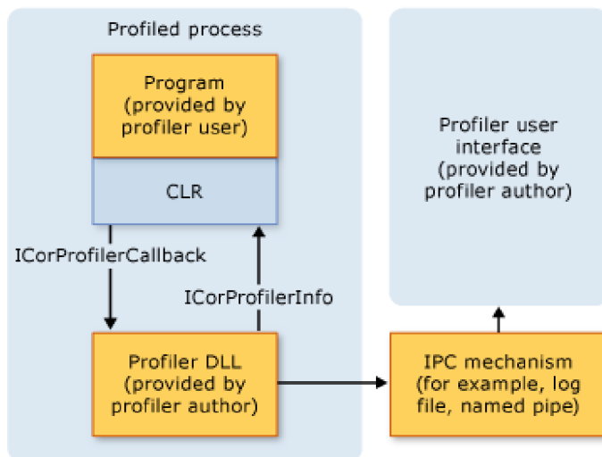
Obrázek 5.3: Schématická ilustrace profileru DLL spolupracujícího s profilovaným programem a CLR [24].
