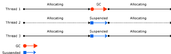
Obrázek 5.2: Ilustrace automatického uvolnění paměti ve vícevláknových programech [21].
