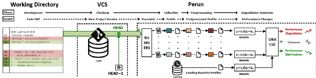
Obrázek 3.2: Ilustrace obvyklého pracovního postupu nástroje Perun. Perun při každé nové verzi naměří nové výkonnostní profily a provede porovnání s předchozími profily. Perun následně provede vyhodnocení optimalizace nebo degradace výkonu projektu [34].
