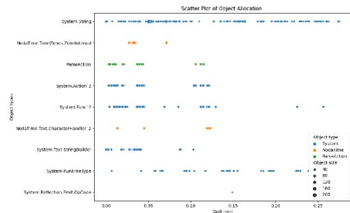
Obrázek 7.3: Bodový graf pro zobrazení alokací objektů daných typů ve Wall čase.
