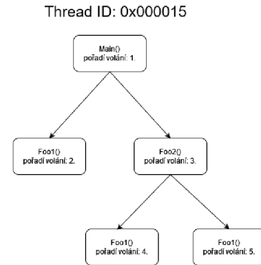
Obrázek 6.3: Ilustrace grafu volání.
