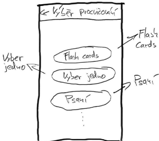
Obrázek 4 – Výběr procvičování
