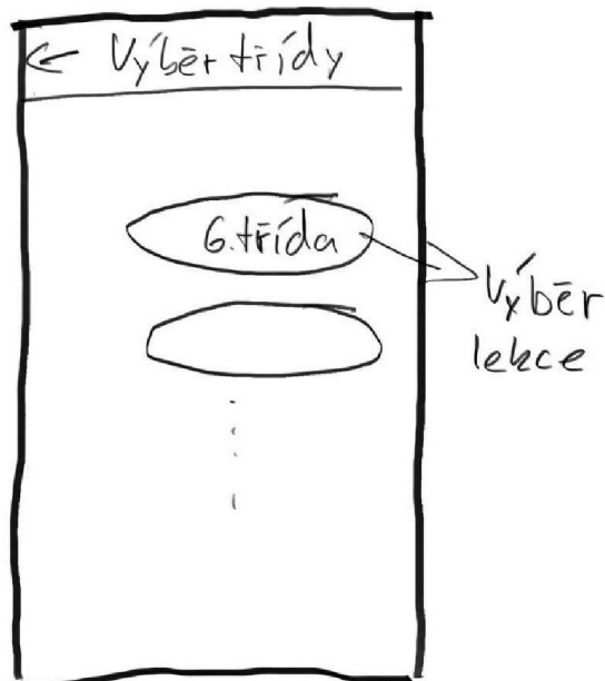
Obrázek 2 – Výběr třídy
