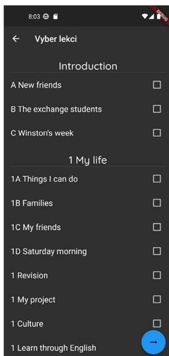
Obrázek 10 – Výběr lekce
