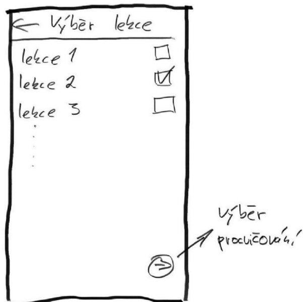
Obrázek 3 – Výběr lekce
