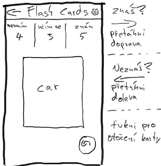
Obrázek 5 – Flash cards
