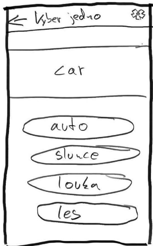
Obrázek 6 – Vyber jedno
