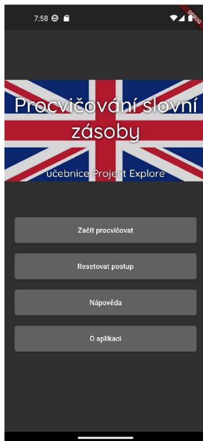
Obrázek 8 – Domovská obrazovka
