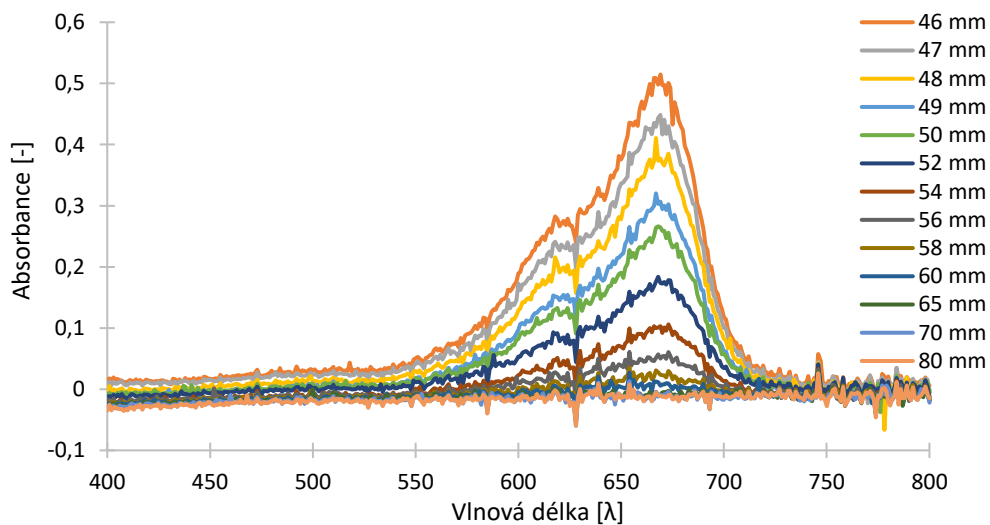
Obrázek 38: Absorpční spektrum gellanového hydrogelu v prostředí deionizované vody s 0,01 g/l MM po 48 hod po korekcí na baselinu .
