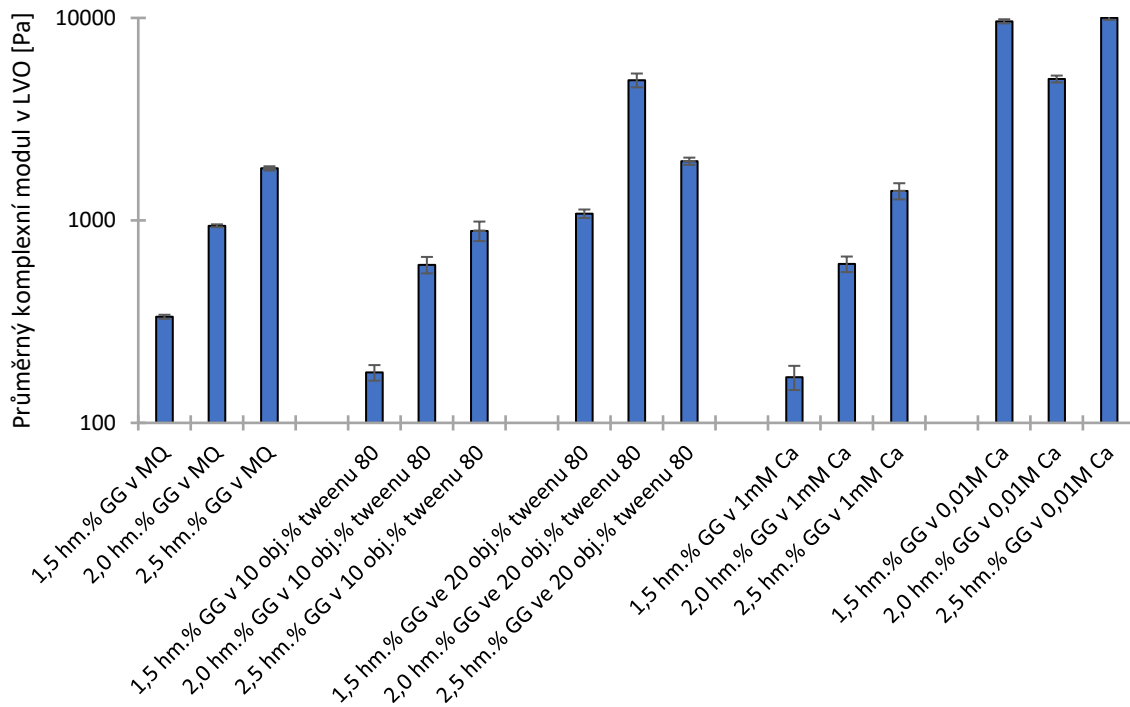
Obrázek 25: Komplexní moduly gellanových hydrogelů.
