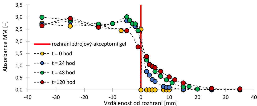
Příloha 16: Časový vývoj koncentračních profilů gellanových hydrogelů v prostředí roztoku 1 mM \text{Ca}^{2+} iontů a MM o koncentraci 0,01 g/l.
