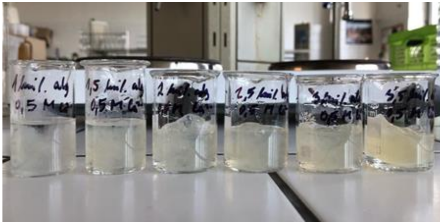
Příloha 4: Koncentrační řada alginátových hydrogelů s 0,5 M \text{CaCl}_2 \cdot 2\text{H}_2\text{O} v poměru 2:1.
