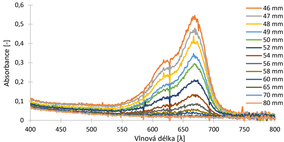
Obrázek 37: Absorpční spektrum gellanového hydrogelu v prostředí deionizované vody s 0,01 g/l MM po 48 hod před korekcí na baselinu .
