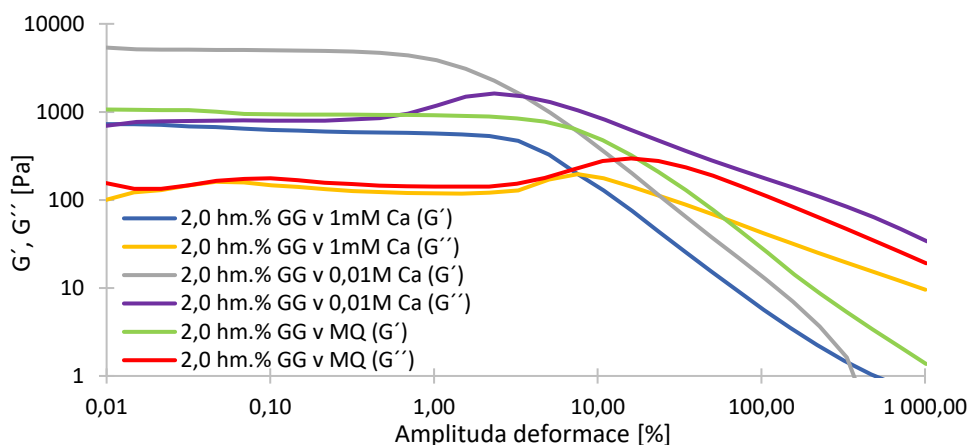
Obrázek 23: Závislost elastických a viskózních modulů 2,0 hm. % gellanových hydrogelů v prostředí deionizované vody a v prostředí roztoků Ca^{2+} iontů na amplitudě deformace.
