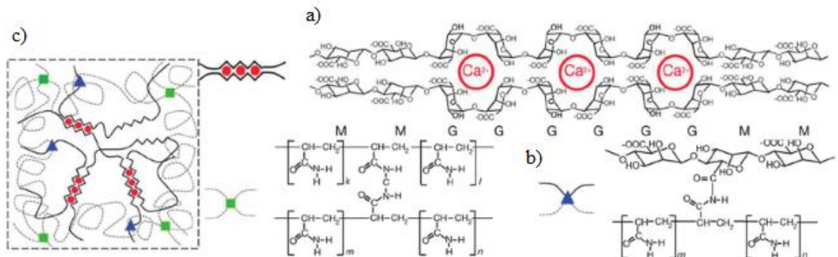
Obrázek 3: a) Struktura alginátu, b) Struktura polyakrylamidu, c) Struktura hybridního hydrogelu [7].
