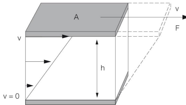
Obrázek 4: Model paralelních desek [9].
