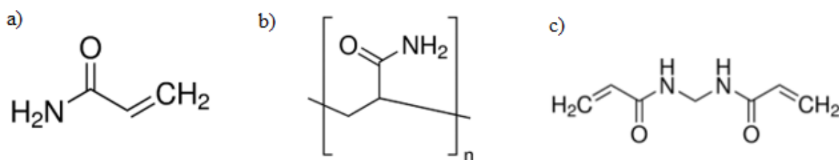
Obrázek 12: Chemická struktura a) akrylamidu, b) polyakrylamidu, c) \text{N,N}' –metylenbisakrylamidu [29].
