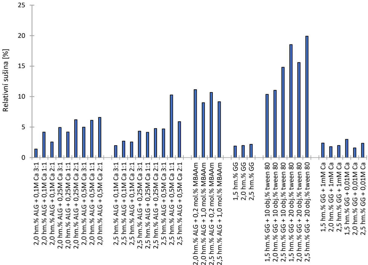
Obrázek 19: Hodnoty obsahů relativních sušín všech připravených hydrogelů.
