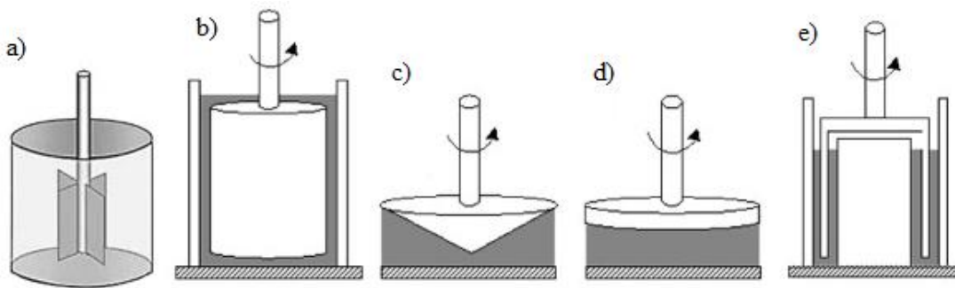
Obrázek 7: Měřící systémy rotačního reometru a) lopatky, b) válec–válec, c) kužel–deska, d) deska–deska, e) double-gap [14].
