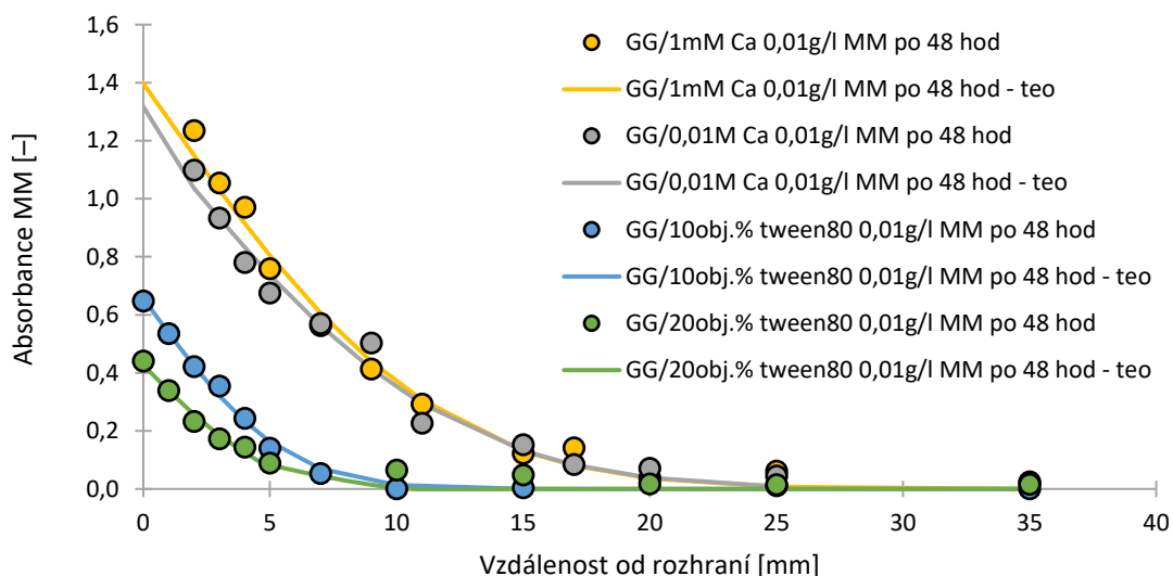
Obrázek 45: Nafitované koncentrační profily pro difúzi akceptorních gellanových hydrogelů s 0,01 g/l MM v prostředí 1 mM a 0,01 M roztoku Ca^{2+} iontů a 10 obj. % a 20 obj. % roztoku tweeku 80.
