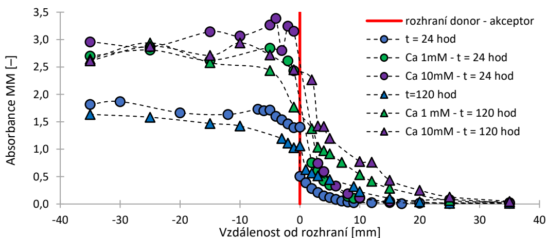
Příloha 20: Koncentrační profily gellanových hydrogelů s MM o koncentraci 0,01 g/l v prostředí 1 mM Ca 2+ a 0,01 M Ca 2+ po 24 a 120 hod.
