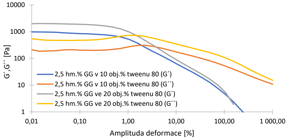
Příloha 7: Závislost elastických a viskózních modulů 2,5 hm. % gellanových hydrogelů v prostředí tweenu 80 na amplitudě deformace.
