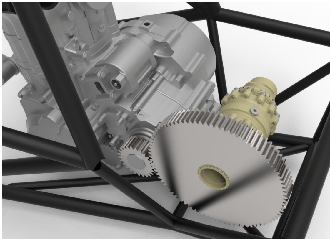
Obr. 9 Navrhnuté čelné ozubené súkolesie umiestnené v ráme spolu s motorom a diferenciálom
