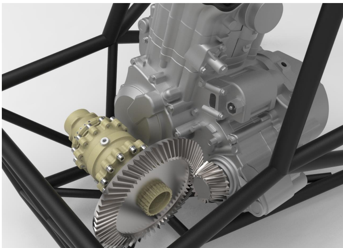
Obr. 11 Navrhnuté kužeľové ozubené súkolesie so šikmými zubmi umiestnené v ráme spolu s motorom a diferenciálom
