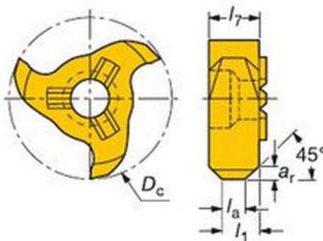
Obr.13 CoroMill 327. [17]
