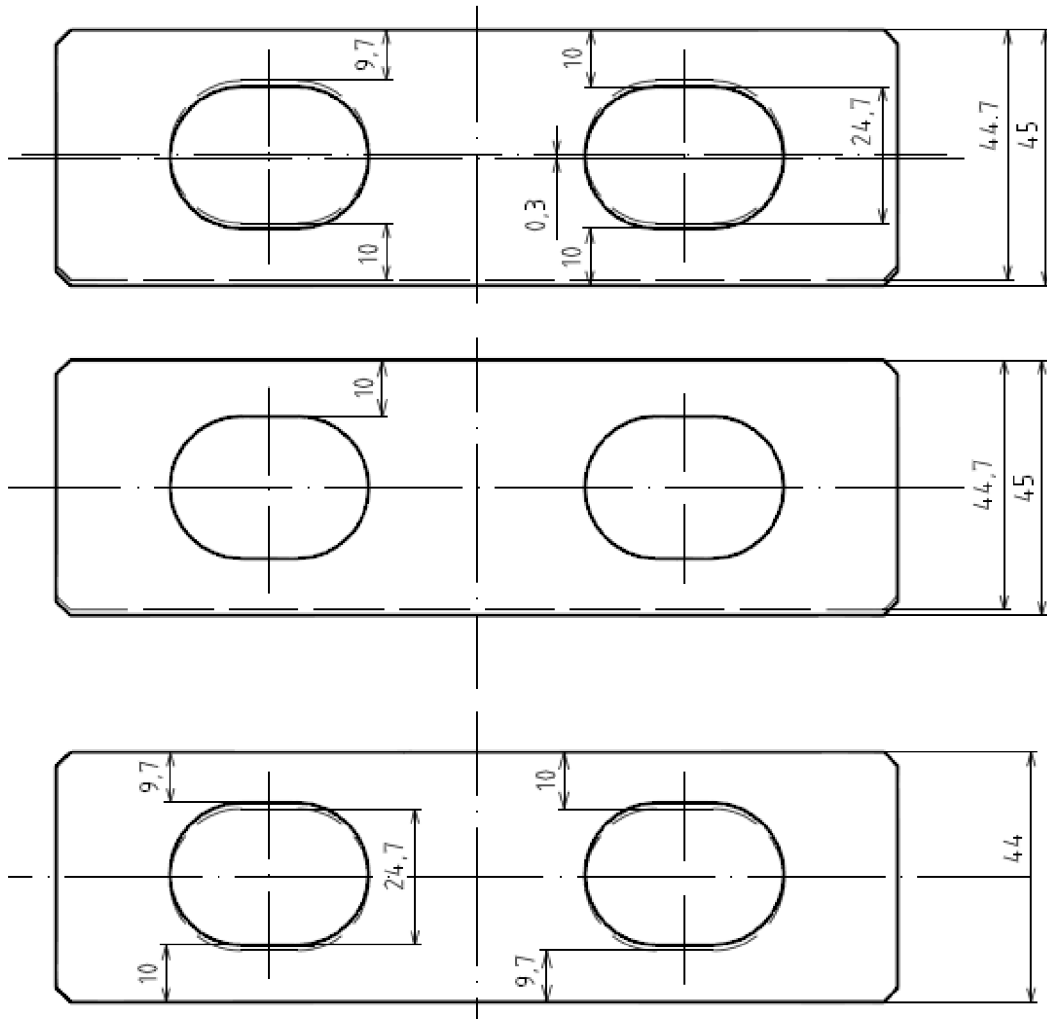
Obr. 15 Znáozornenie tolerančnej chyby pri umiestnení v prípravku.
