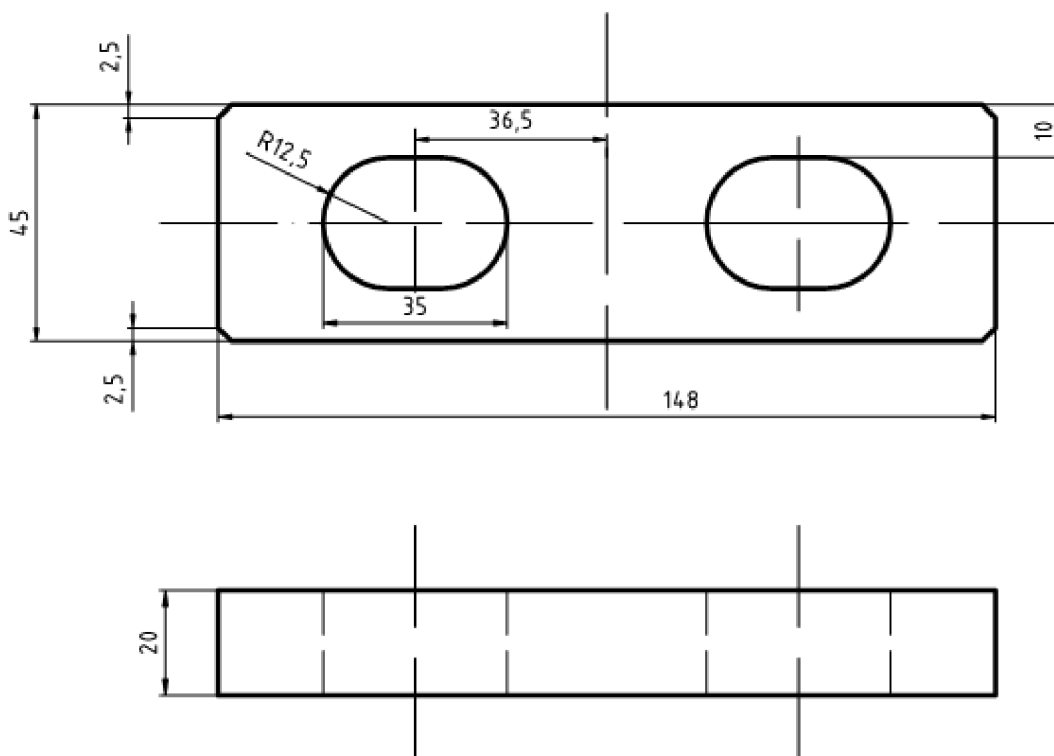
Obr.14 Tvar a rozmery obrobku.
