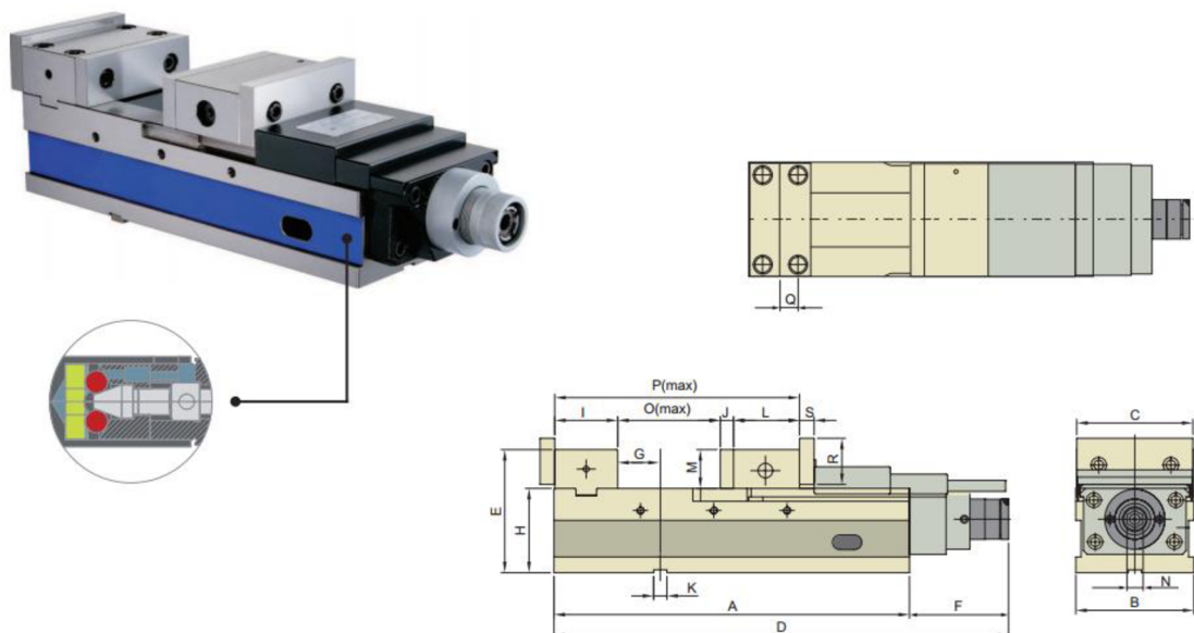
Obr. 1 MC Mechanický zverák AVQ - 100, 125, 160, 200 G/HV. [2]
