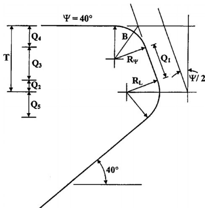
Obr. 22 Lineárně tvořený model [34]
