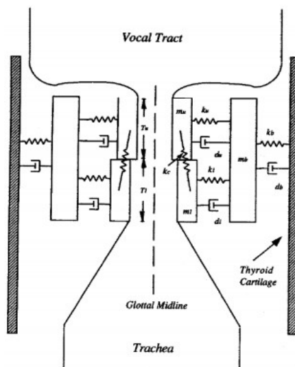
Obr. 15 Tříhmotový model [3]
