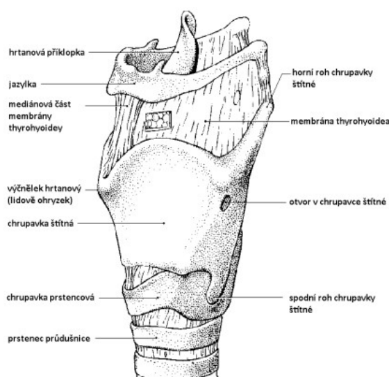
Obr. 4 Kostra hrtanu [9]
