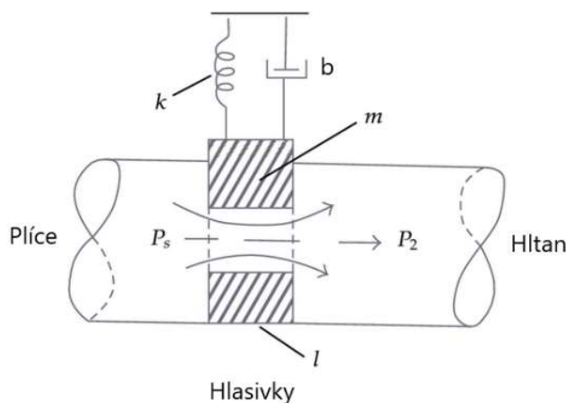
Obr. 13 Jednohmotový model [44]
