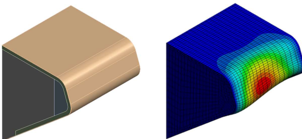
Obr. 42 vlevo původní tvar modelu; vpravo 3. vlastní tvar pro úhel 40^\circ
