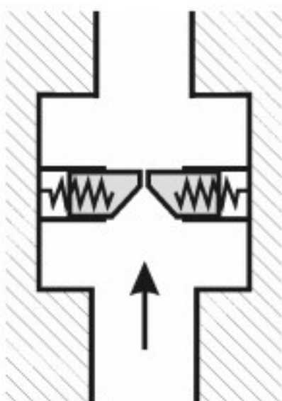
Obr. 12 Ewaldova píšťala [3]
