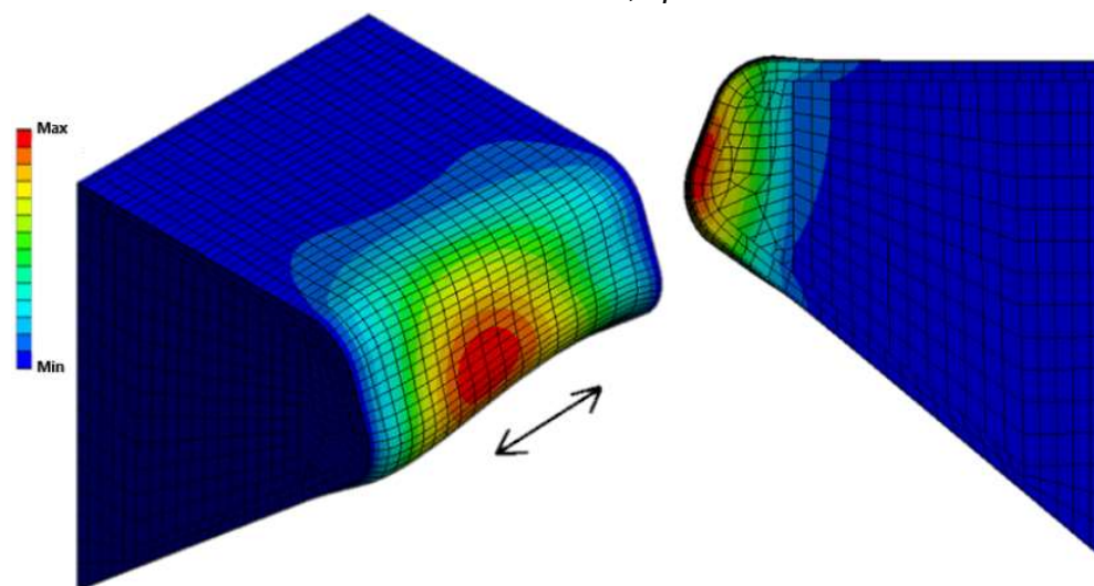
Obr. 46 vlevo model 3. vlastní frekvence úhlu +40^\circ ; vpravo řez v místě maximální deformace
