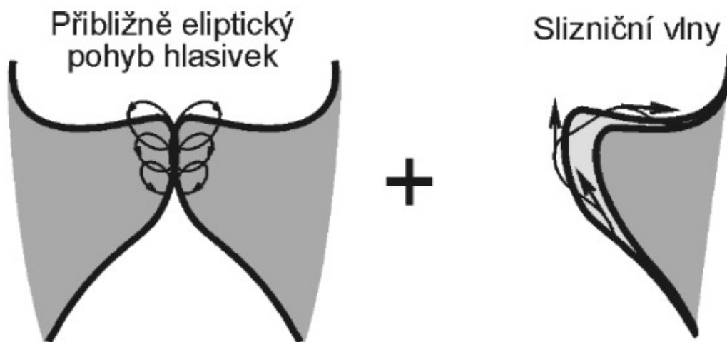
Obr. 9 Pohyby hlasivek [22]
