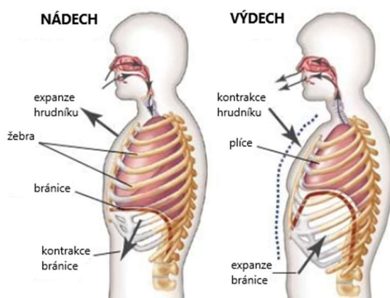
Obr. 3 Mechanika dýchání [42]
