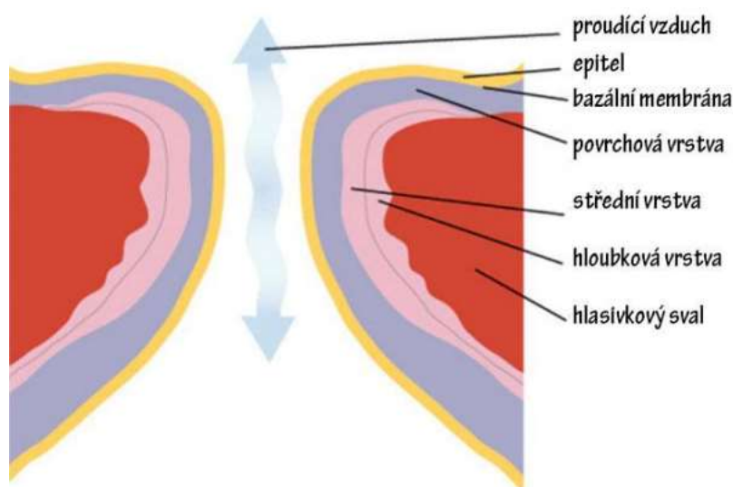
Obr. 7 Řez hlasivkami [11]
