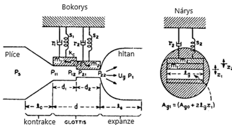
Obr. 14 Dvouhmotový model [3]
