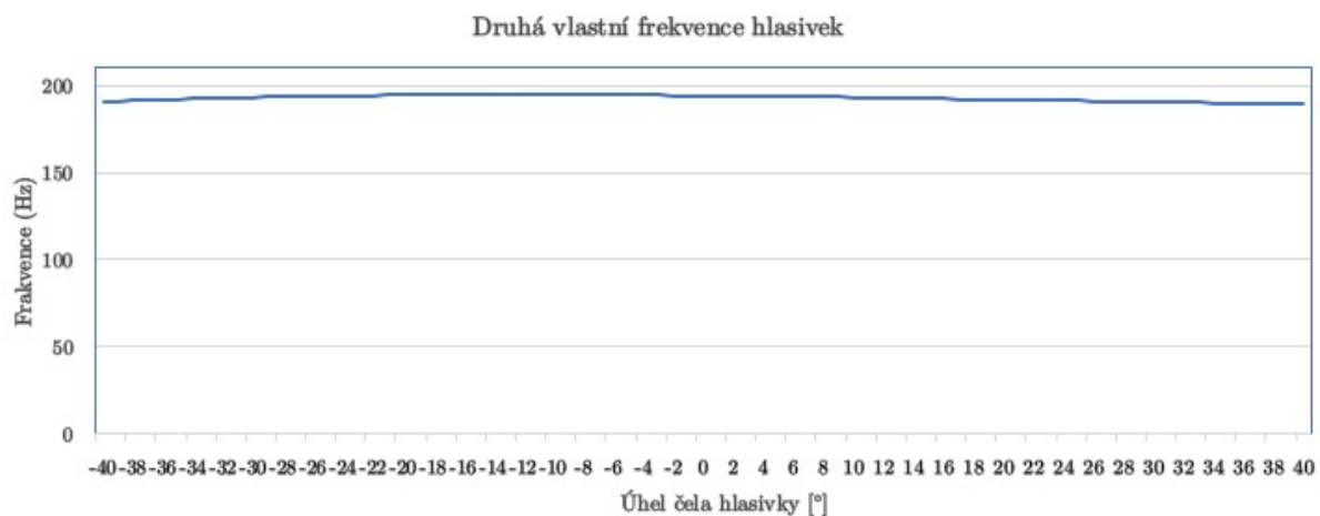
Obr. 33 Graf druhé vlastní frekvence hlasivek
