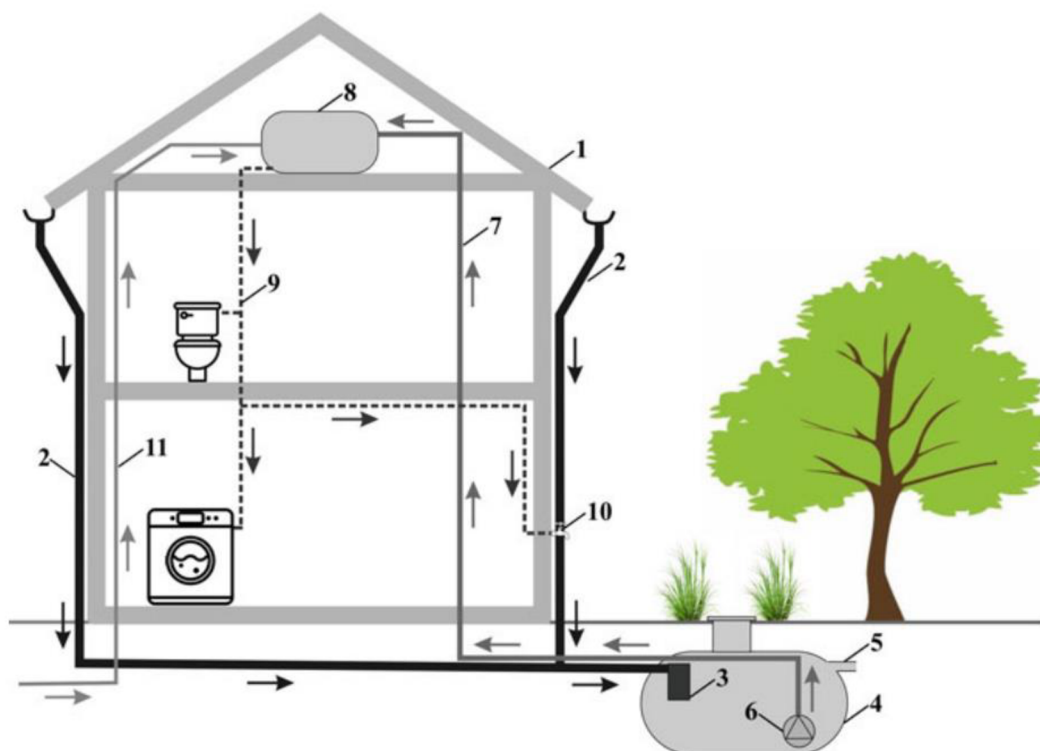
Obr. 9 Schéma systému zachycování dešťové vody (Sly's 2013)
