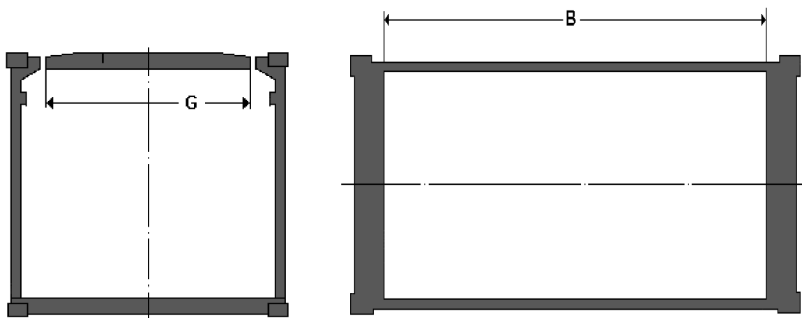
Obr. 34 Otvor v Hard-top kontajneroch [38]
