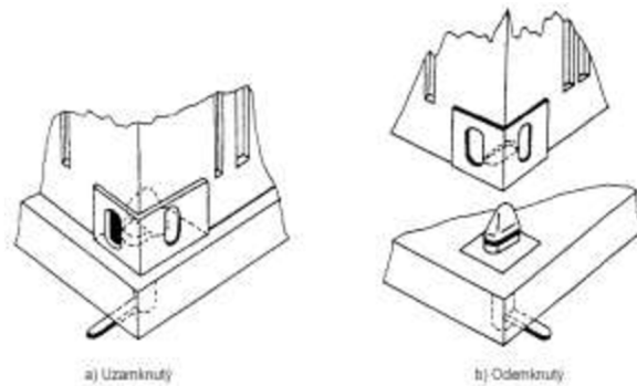
Obr. 51 Otočný zámok na návесе [49]
