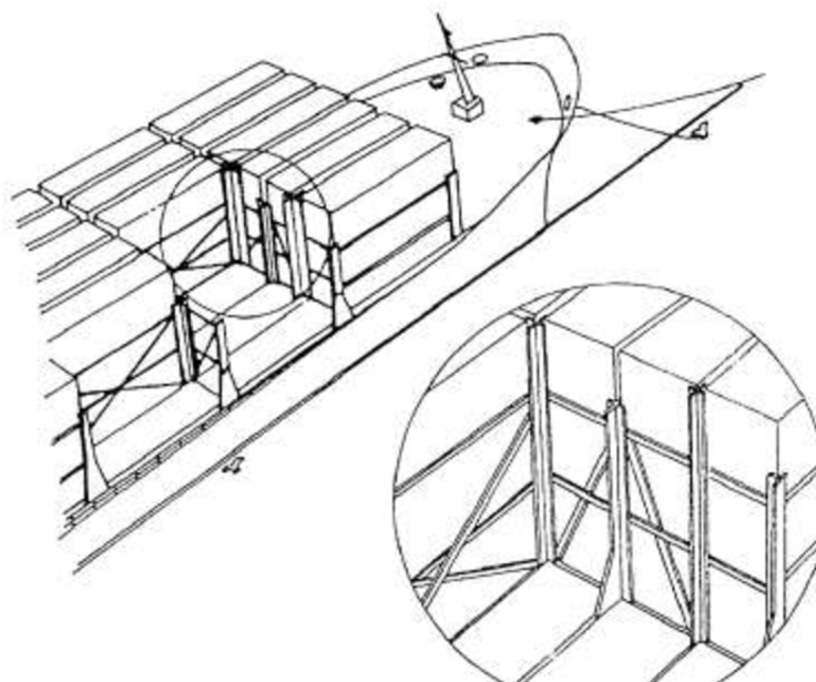
Obr. 42 Vodička na lodi [49]
