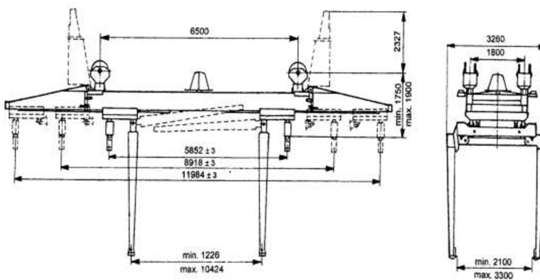
Obr. 56 Kombinovaný spreader[26]
