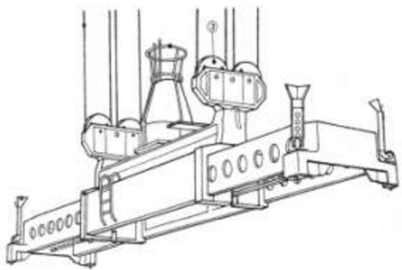
Obr. 55 Automatický spreader[26]
