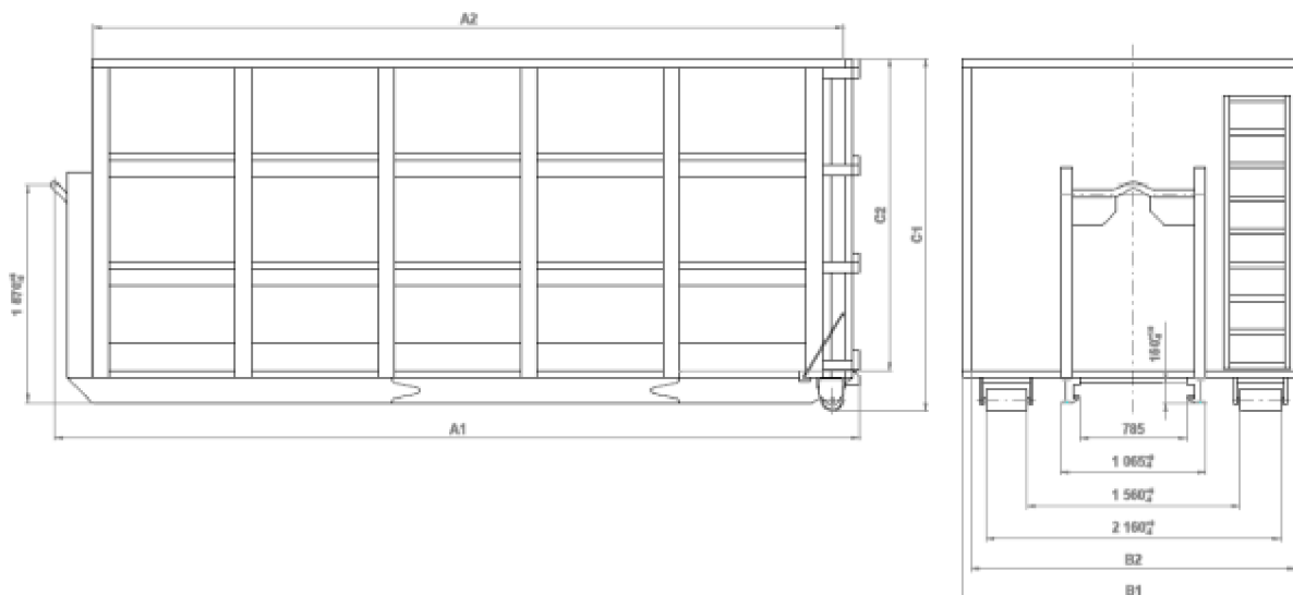
Obr. 7 vaňový kontajner podľa DIN 30 722 [18]
