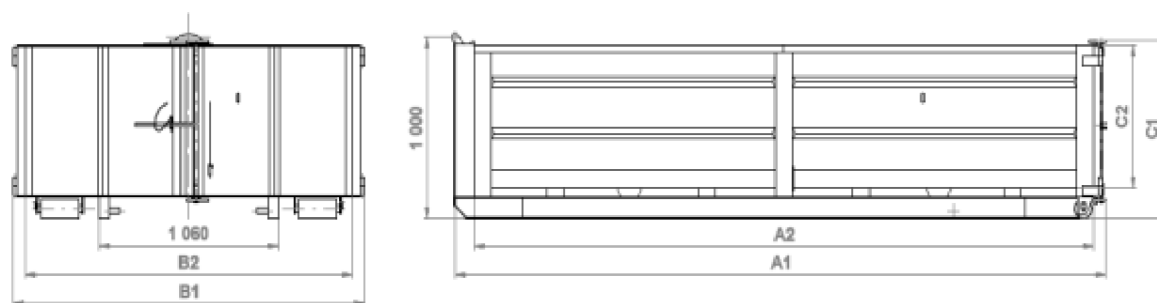
Obr. 8 Vaňový kontajner [19]
