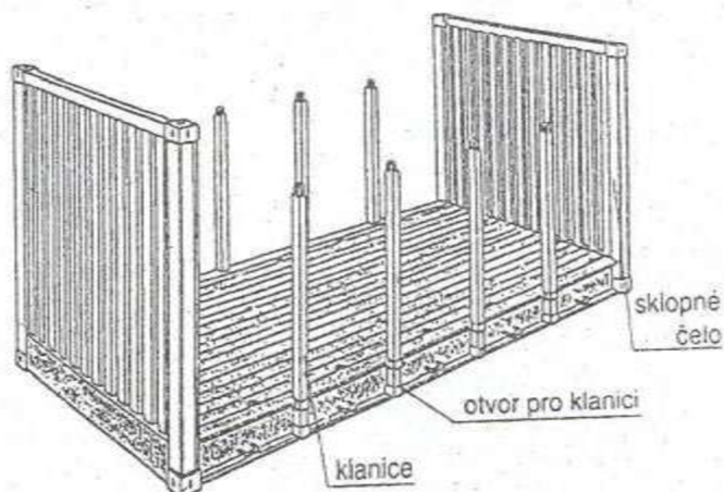
Obr. 38 Plošinový kontajner[42]
