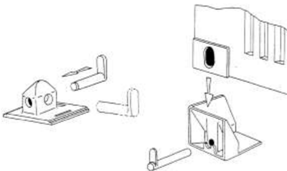
Obr. 50 Prvky na zabezpečenie kontajera [49]
