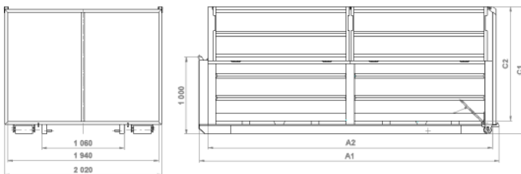
Obr. 13 Veľkoobjemový kontajner so sklupnými bočnicami [22]
