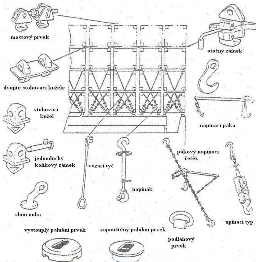
Obr. 44 Fixačné zariadenia [42]
