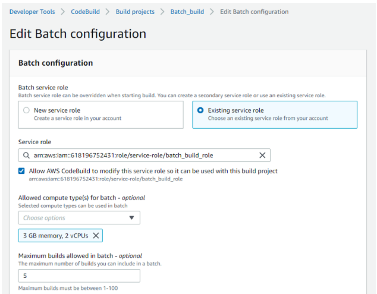
Obrázek 11.10: Nastavení možnosti batch
