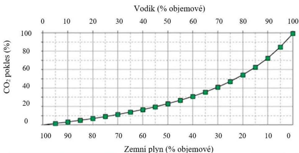
Obr. 15: Vliv množství vodíku v palivu na emisii CO 2 , převzato z [45].
