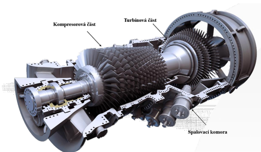
Obr. 4: Základní komponenty plynové turbíny, převzato a upraveno z [5].
