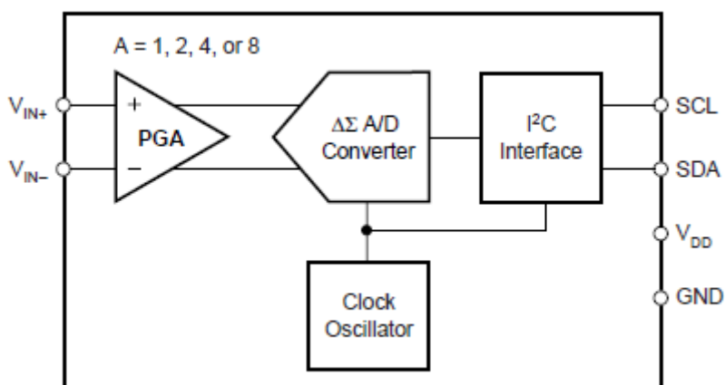
Obr. 4.1. Blokové schéma A/D převodníku ADS1100, převzato z [6].
