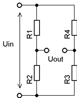
Obr. 1.5. Zapojení Wheatstonova můstku.
