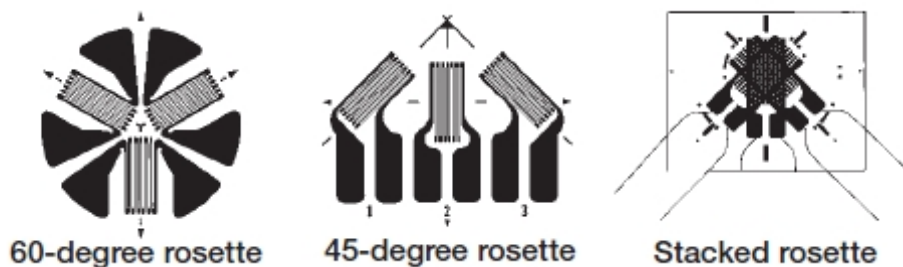
Obr. 1.3: Příklady tříprvkových sdužených tenzometrů, převzato z [9].
