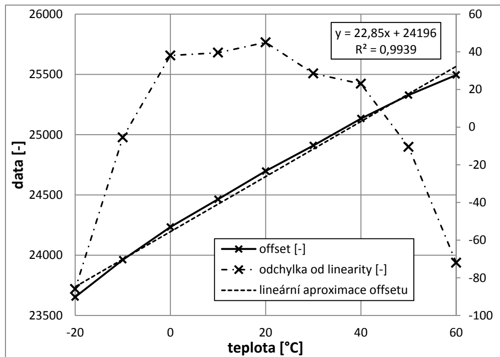
Obr. 8.2: Teplotní závislost offsetu zařízení pro měření s exponenciální kumulací.
