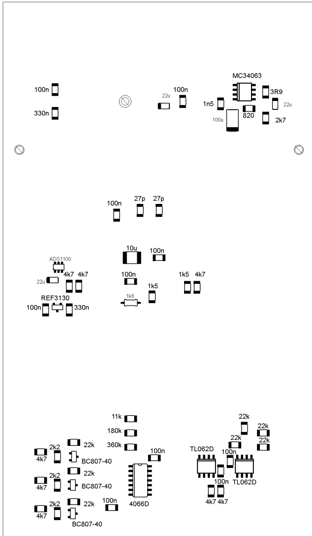
DPS – osazovací plán, strana spojů
