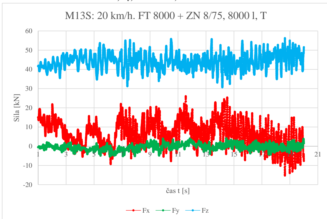
Příloha 11: Graf závislosti sil F_x , F_y , F_z na čase, měření M13S.
