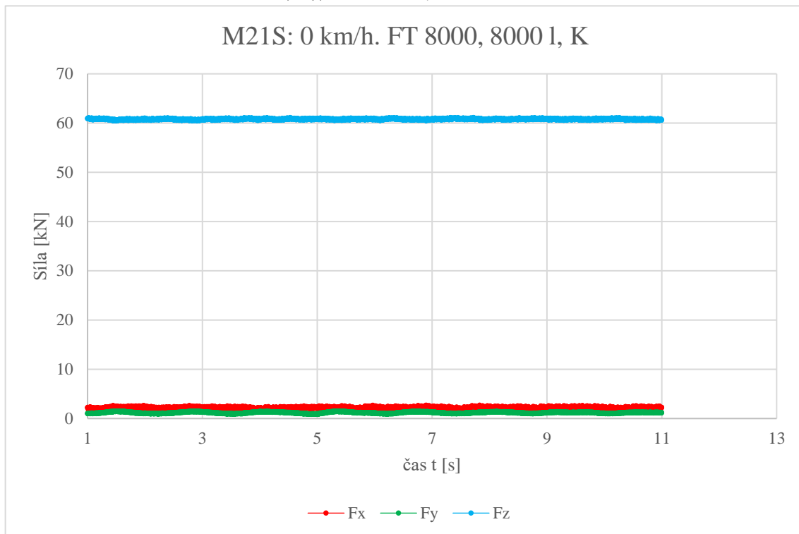
Příloha 17: Graf závislosti sil F_x , F_y , F_z na čase, měření M21S.
