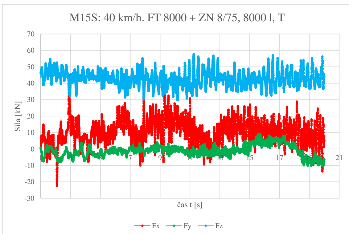
Příloha 12: Graf závislosti sil F_x , F_y , F_z na čase, měření M15S.
