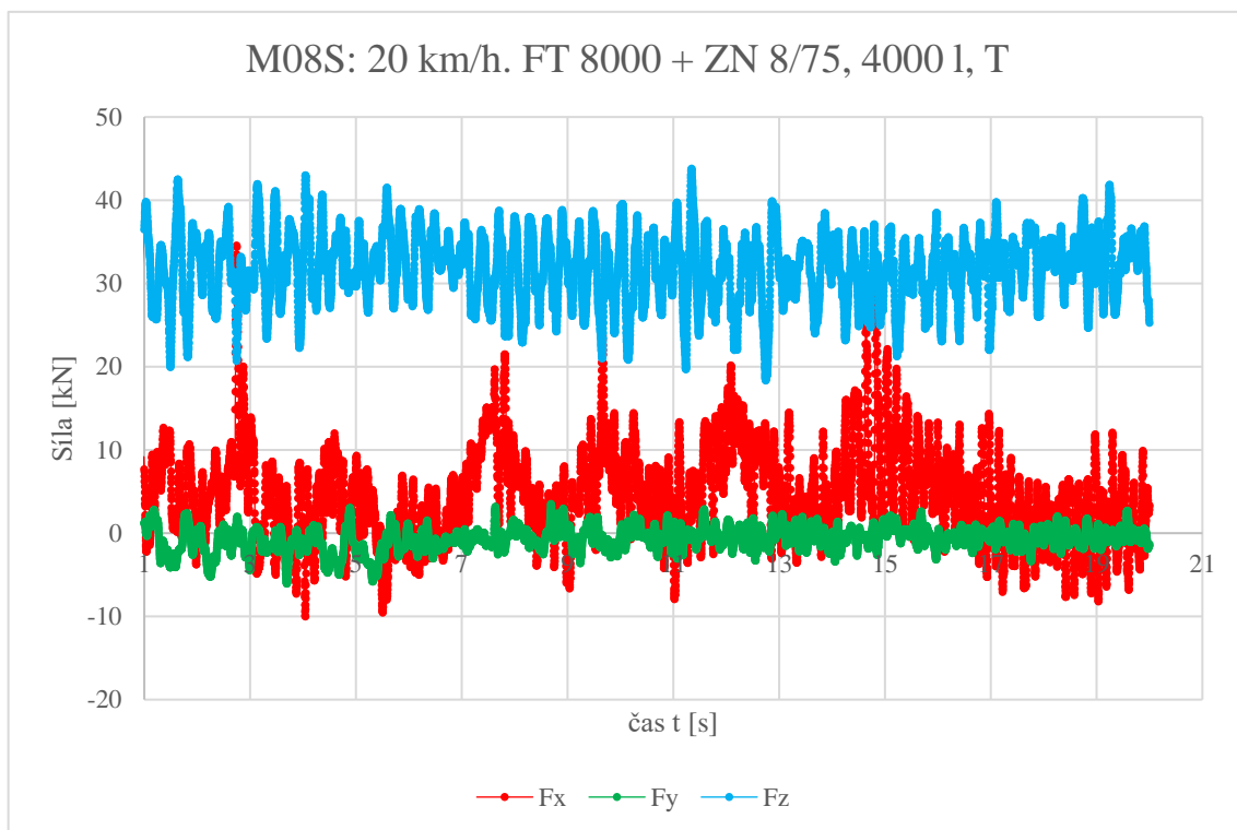
Příloha 8: Graf závislosti sil F_x , F_y , F_z na čase, měření M08S.
