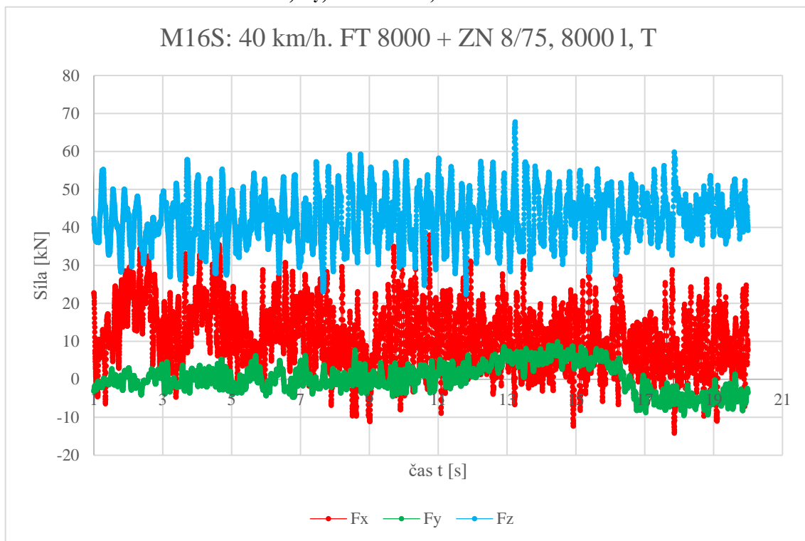
Příloha 13: Graf závislosti sil F_x , F_y , F_z na čase, měření M16S.
