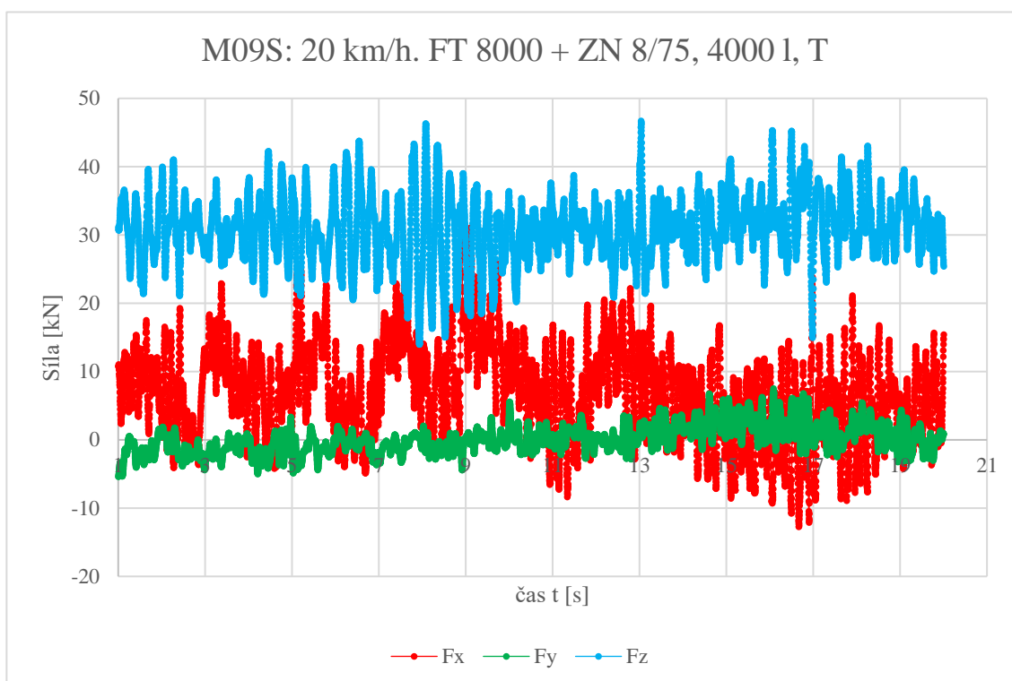
Příloha 9: Graf závislosti sil F_x , F_y , F_z na čase, měření M09S.
