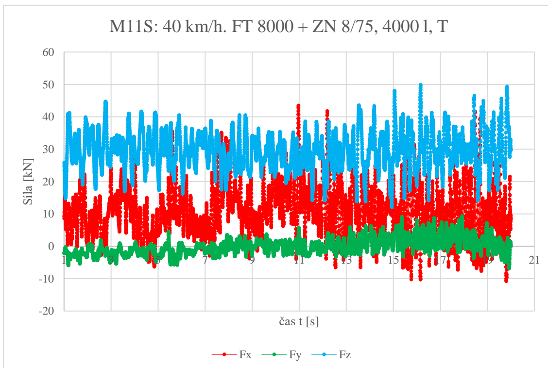
Příloha 10: Graf závislosti sil F_x , F_y , F_z na čase, měření M11S.
