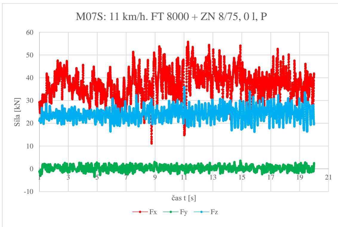
Příloha 7: Graf závislosti sil F_x , F_y , F_z na čase, měření M07S.
