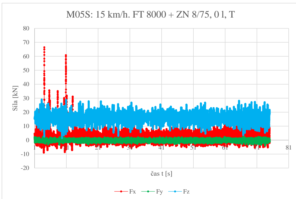
Příloha 5: Graf závislosti sil F_x , F_y , F_z na čase, měření M05S.
