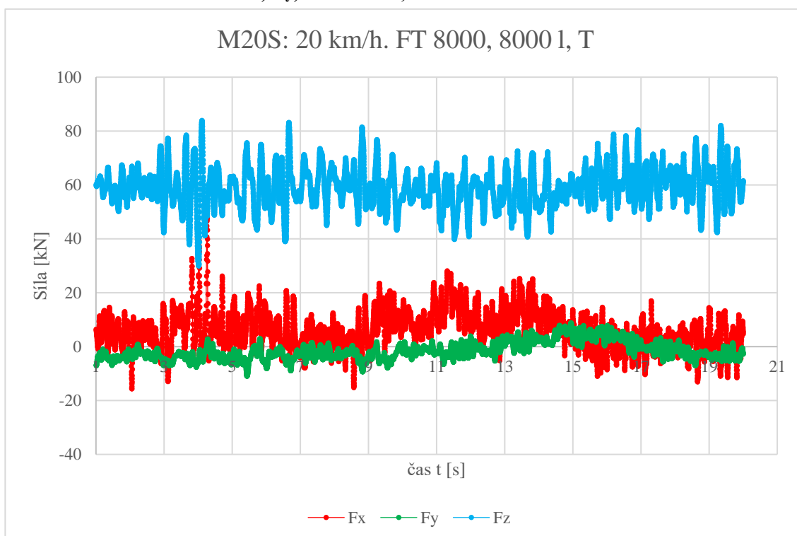
Příloha 16: Graf závislosti sil F_x , F_y , F_z na čase, měření M20S.
