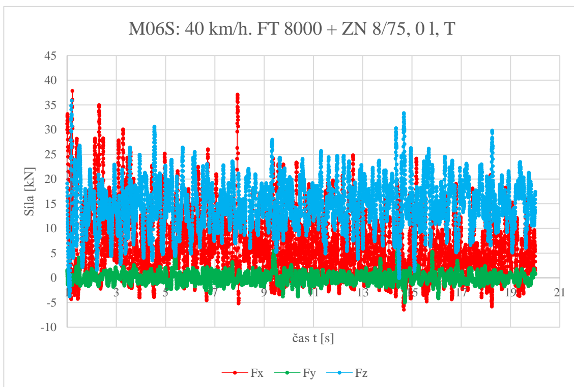
Příloha 6: Graf závislosti sil F_x , F_y , F_z na čase, měření M06S.
