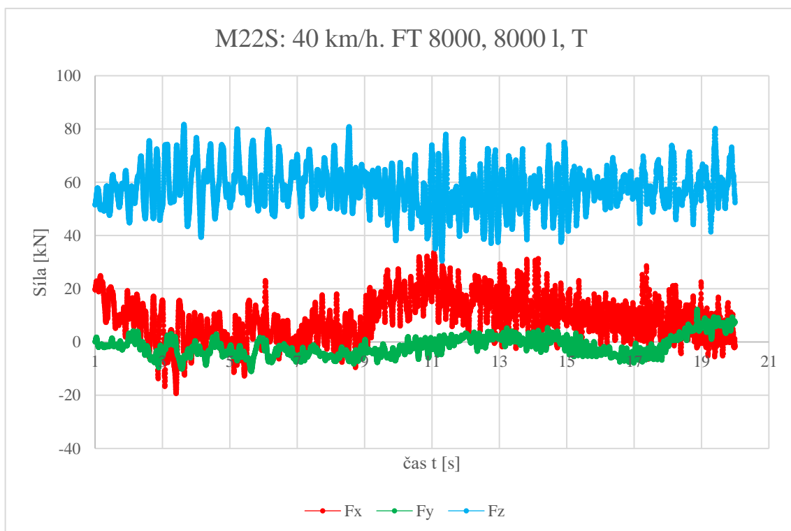
Příloha 18: Graf závislosti sil F_x , F_y , F_z na čase, měření M22S.
