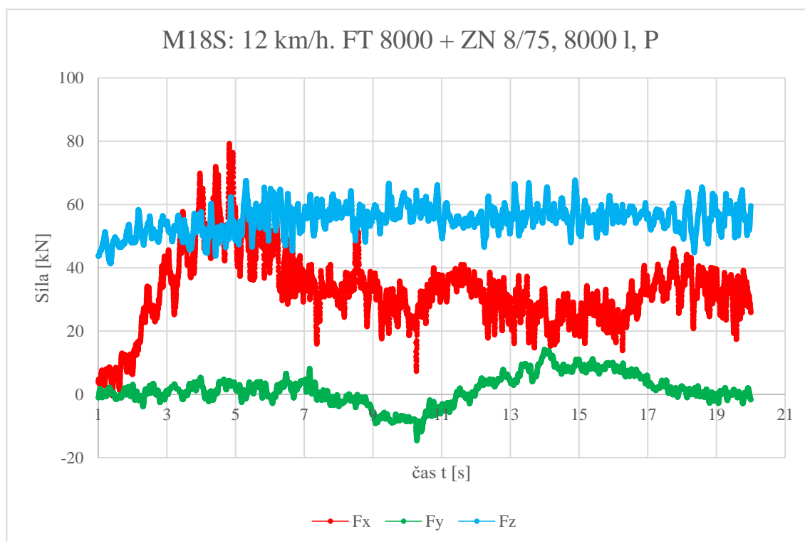
Příloha 15: Graf závislosti sil F_x , F_y , F_z na čase, měření M18S.
