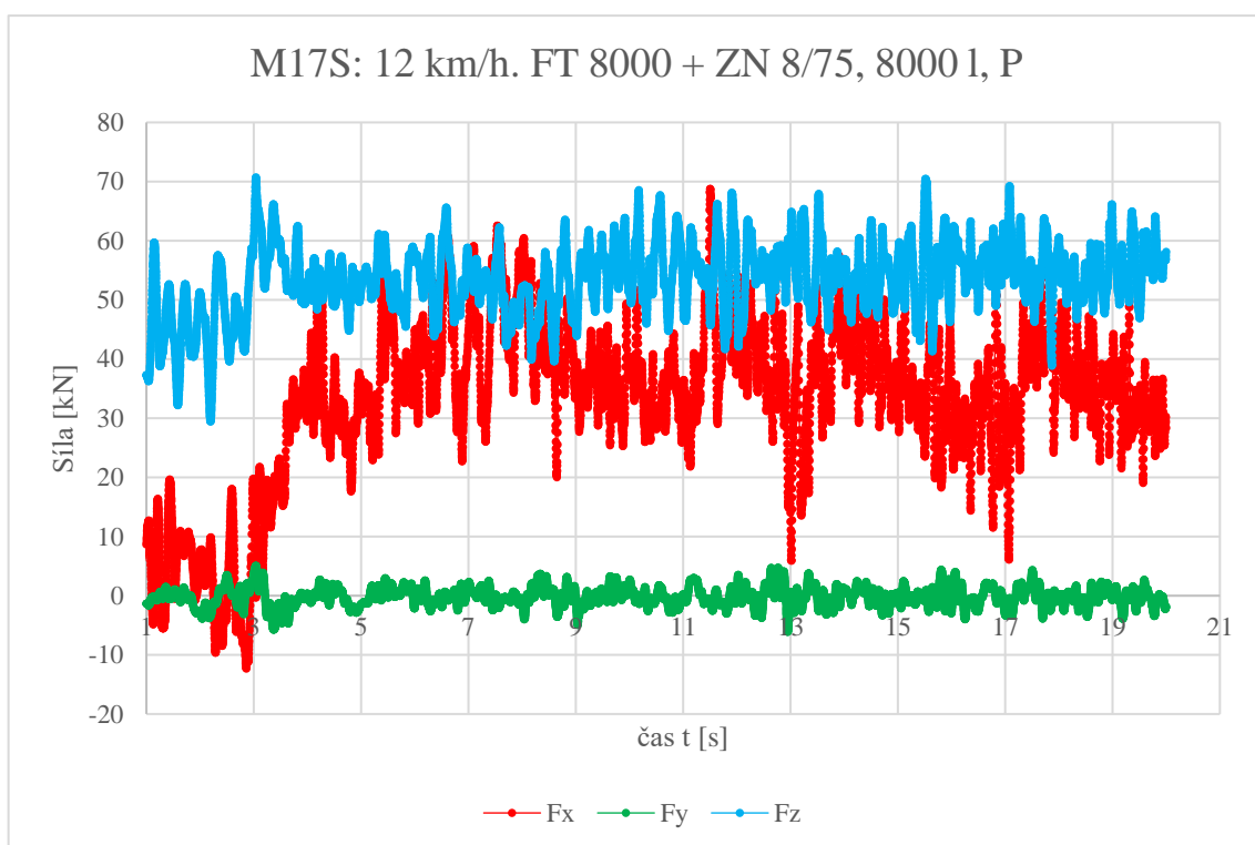
Příloha 14: Graf závislosti sil F_x , F_y , F_z na čase, měření M17S.
