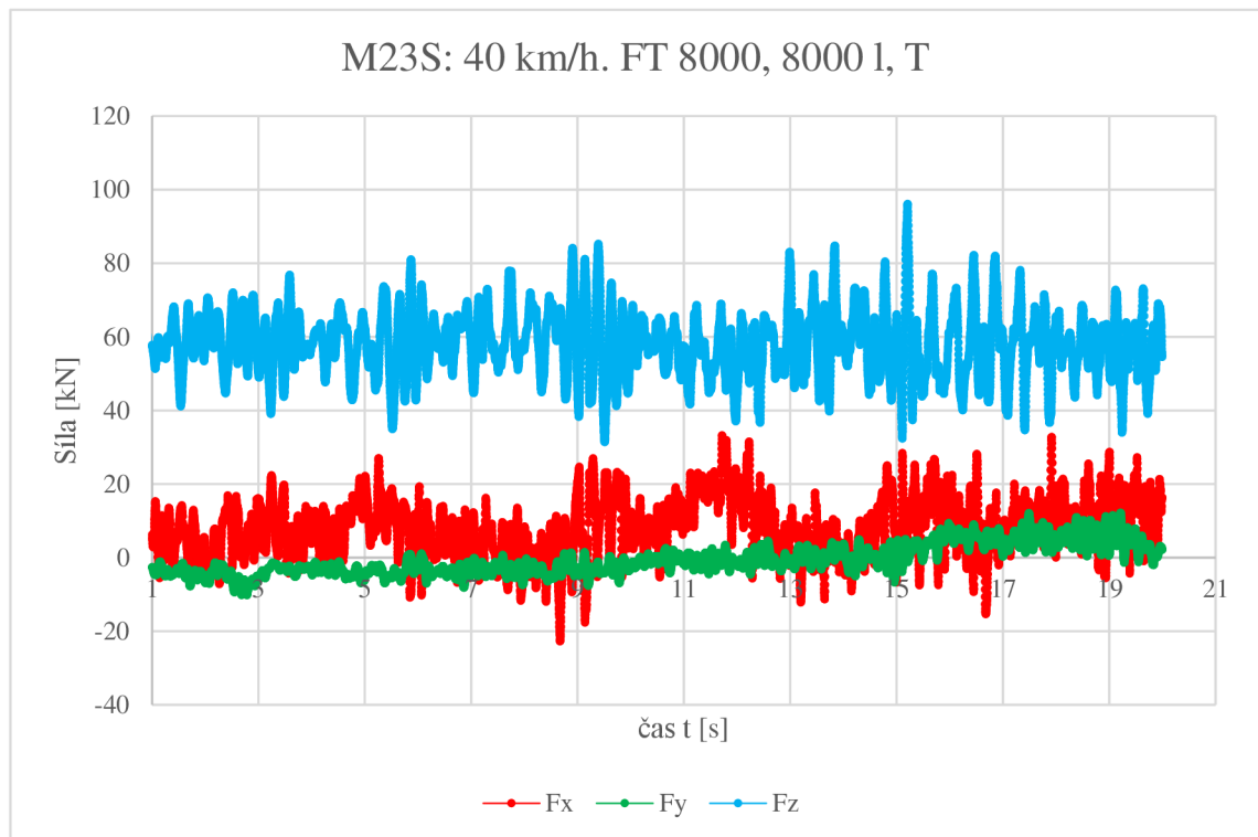
Příloha 19: Graf závislosti sil F_x , F_y , F_z na čase, měření M23S.
