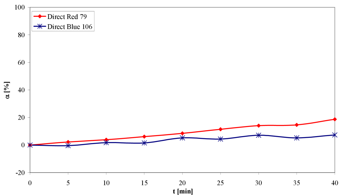
Obr. 10: Srovnání průběhu rozkladu jednotlivých barviv, použitá barviva Direct Blue 106 a Direct Red 79, elektrolyt NaCl, počáteční vodivost G = 500 \mu\text{S}\cdot\text{cm}^{-1} , P = 30 \text{ W} , katodový prostor
