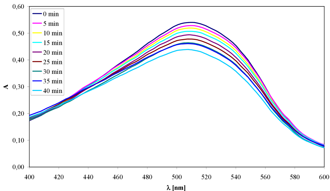
Obr. 14: Vliv elektrolyzy na posun absorpčního maxima, použité barvivo Direct Red 79, elektrolyt NaCl, počáteční vodivost G = 500 \mu\text{S}\cdot\text{cm}^{-1} , P = 30 \text{ W} , katodový prostor
