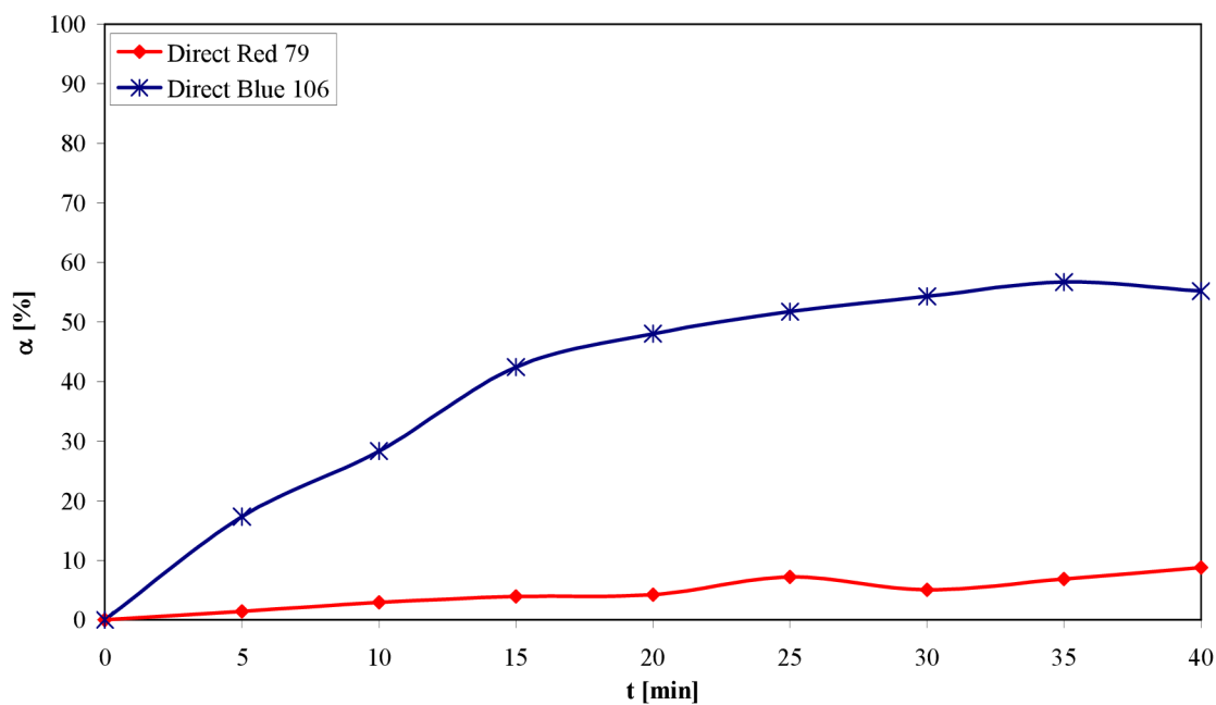
Obr. 9: Srovnání průběhu rozkladu jednotlivých barviv, použitá barviva Direct Blue 106 a Direct Red 79, elektrolyt NaCl, počáteční vodivost G = 500 \mu\text{S}\cdot\text{cm}^{-1} , P = 30 \text{ W} , anodový prostor
