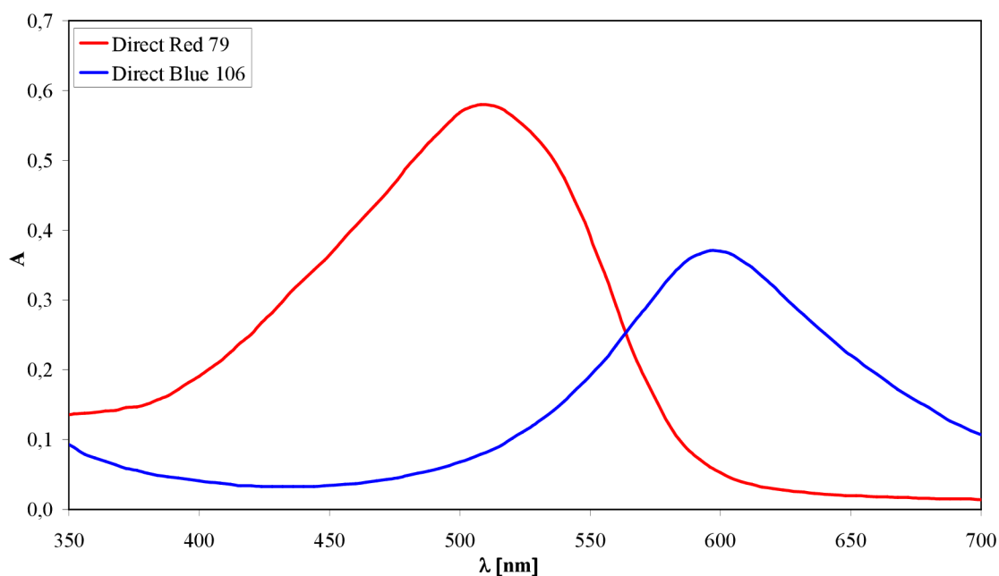
Obr. 6: Absorpční spektra použitých barviv, c_{\text{barviv}} = 15,50 \text{ mol/l}
