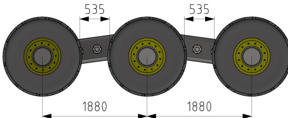
Obr. 5 rozteče kol
