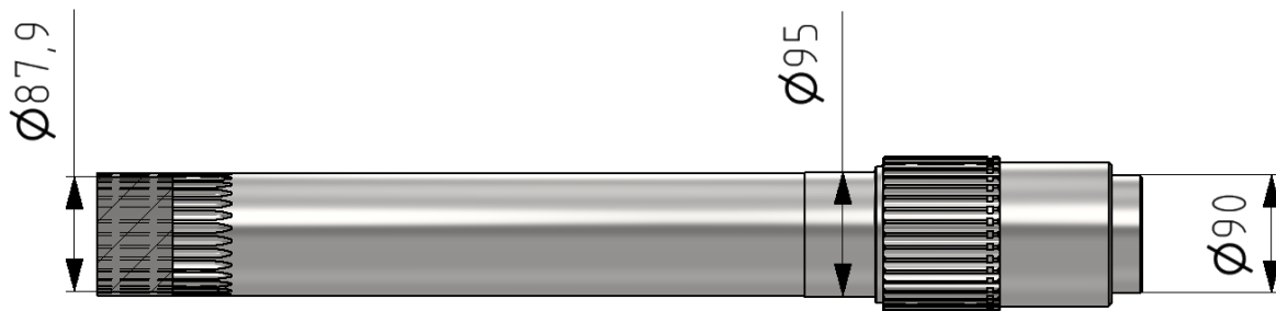
Obr. 12 hřídel pastorku
