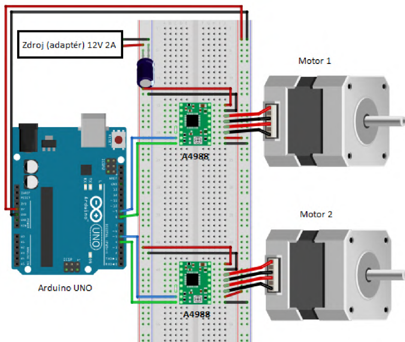
Obr. 4.2: Zapojenie ovládania
