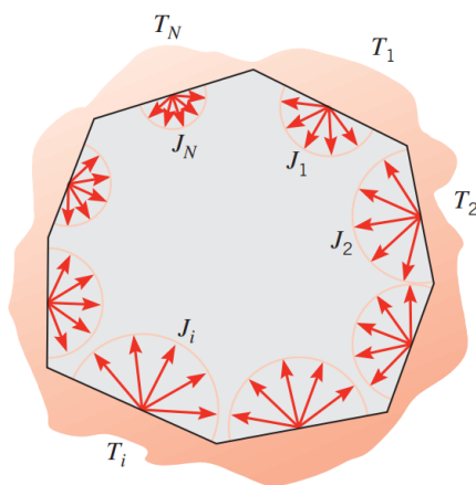
Obrázek 12: Pravidlo součtu [3]
