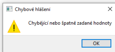
Obrázek 44: Chybové hlášení
