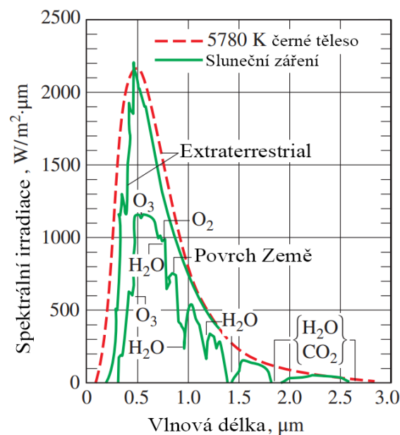
Obrázek 23: Spektrální irradie slunečního záření ([4], upraveno)
