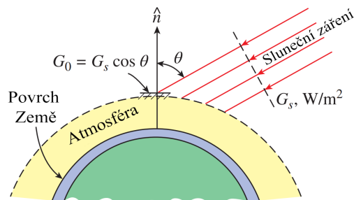
Obrázek 22: Sluneční irradie dopadající na Zemi ([4], upraveno)
