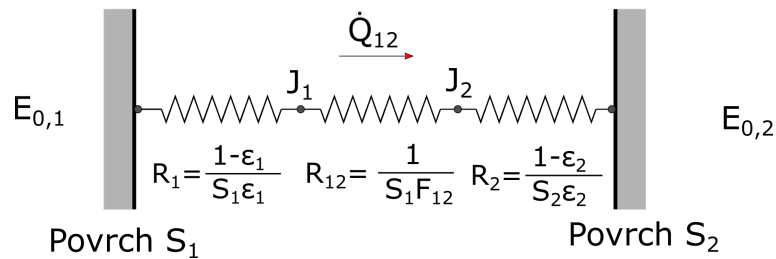
Obrázek 19: Odporové schéma [4]
