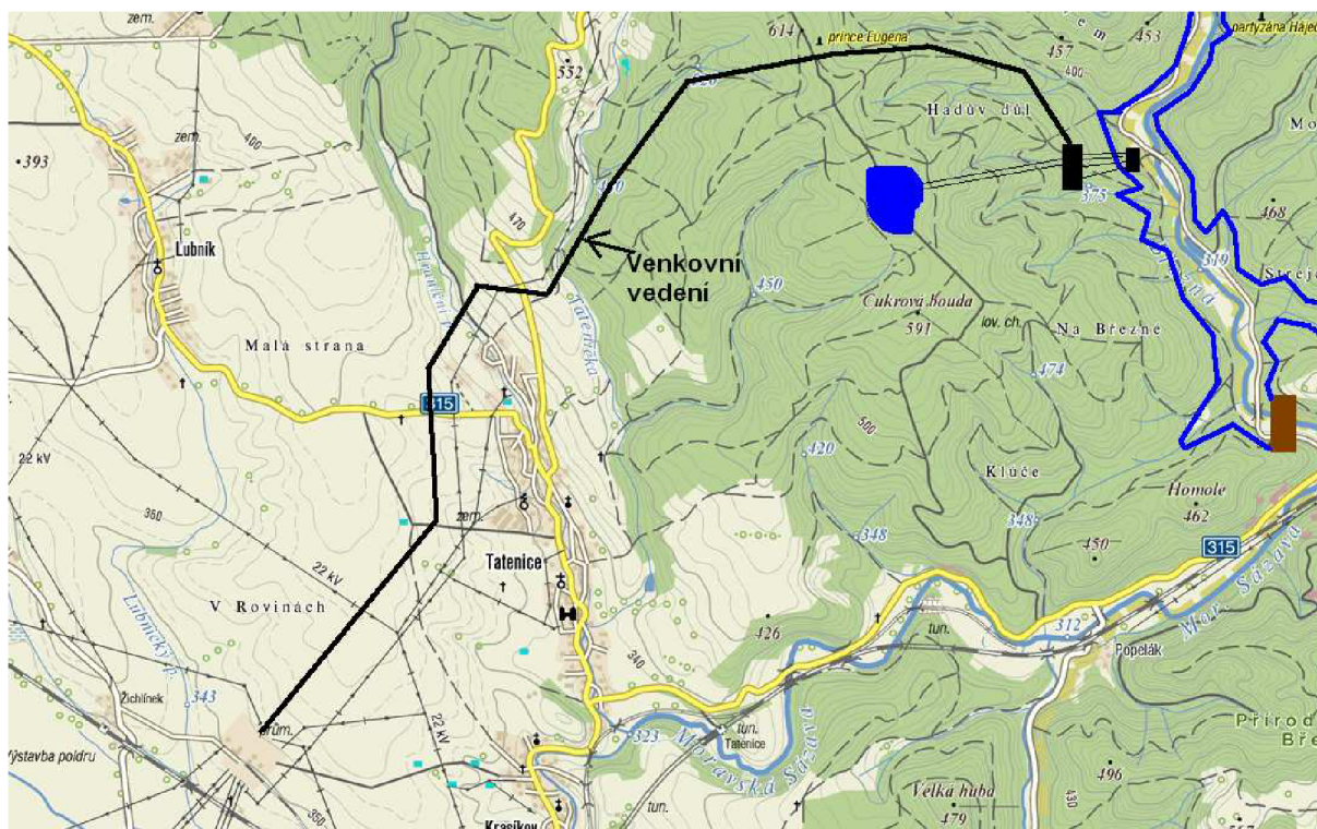
Obr. 5-9 Trasa venkovního vedení vývodu výkonu do rozvodny Krasíkov[12].
