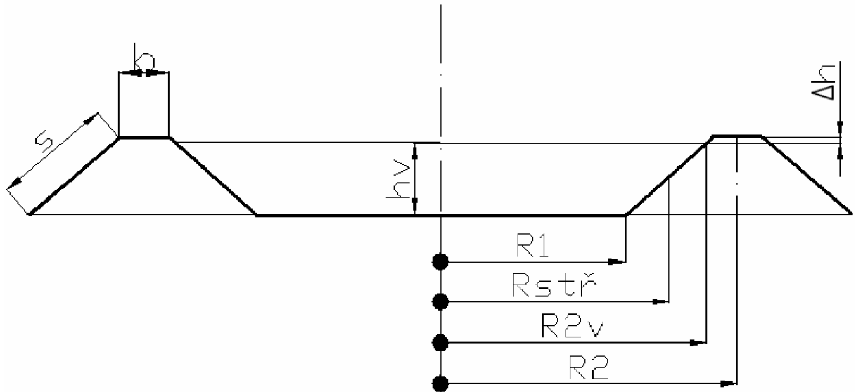
Obr. 5-5 Náčrt horní hráze
