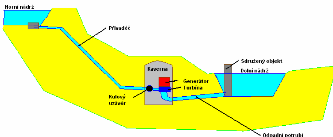
Obr. 3-1 Schéma PVE
