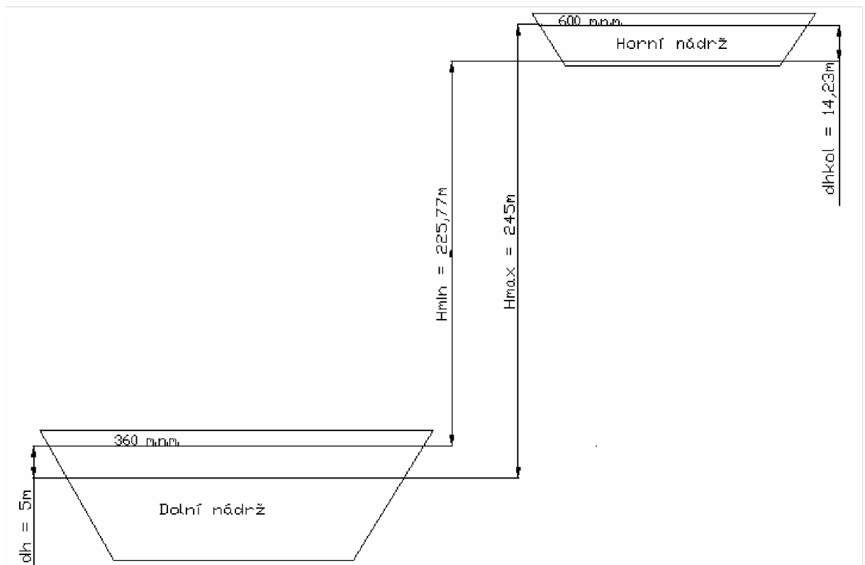
Obr. 5-7 Výškové rozložení nádrží
