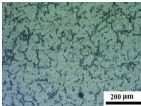
Obrázek 1 Mikrostruktura slitiny AZ61 připravené metodou squeeze casting [8]
