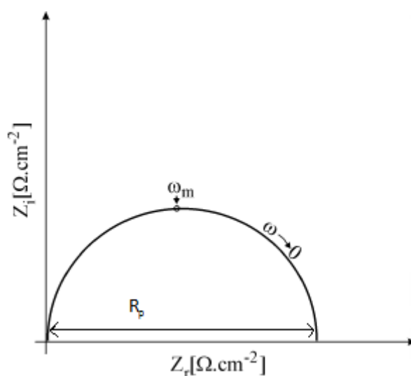
Obrázek 6 Nyquistův diagram [3]
