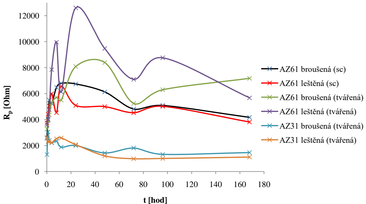
Obrázek 28 Graf závislosti polarizačního odporu na čase
