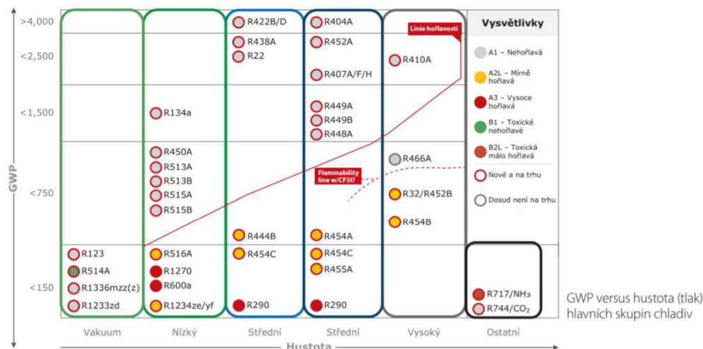
Obrázek 5: Rozdělení chladiv podle vlastností. [27]
