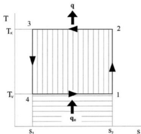
Obrázek 2: T-S diagram levotočivého Carnotova cyklu [6]
