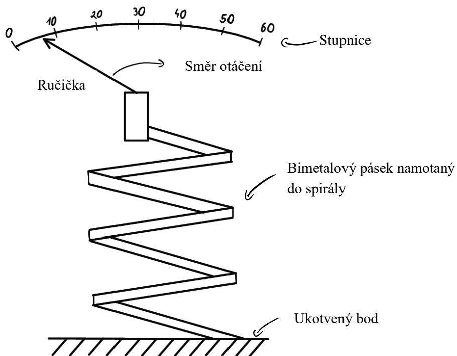
Obrázek 1.3 Konstrukce bimetalového teploměru.
