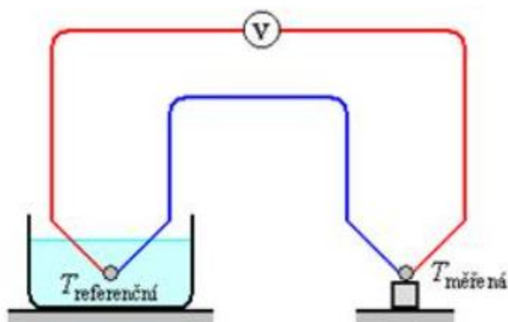
Obrázek 1.13 Princip termočlánku. [9]
