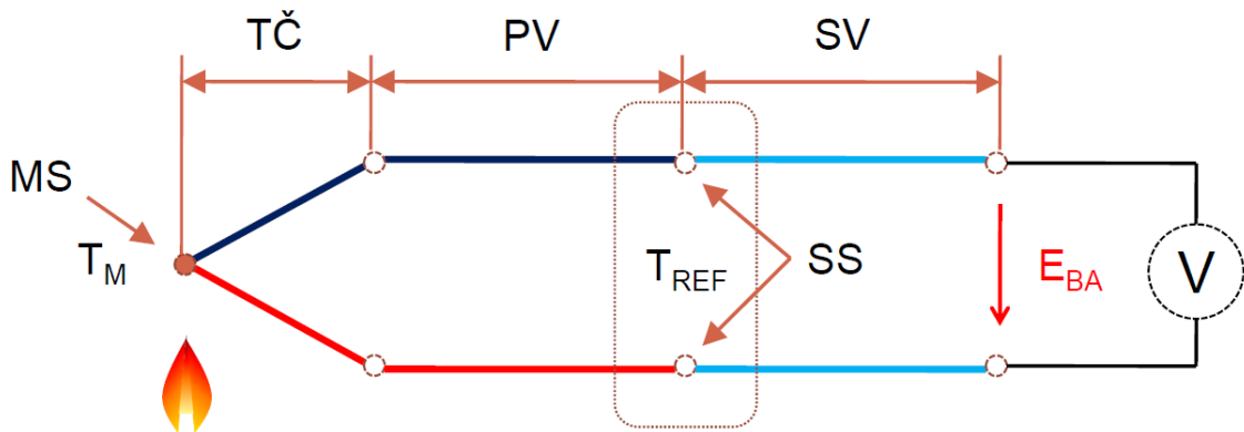
Obrázek 1.15 Schéma termočlánku. [2]
