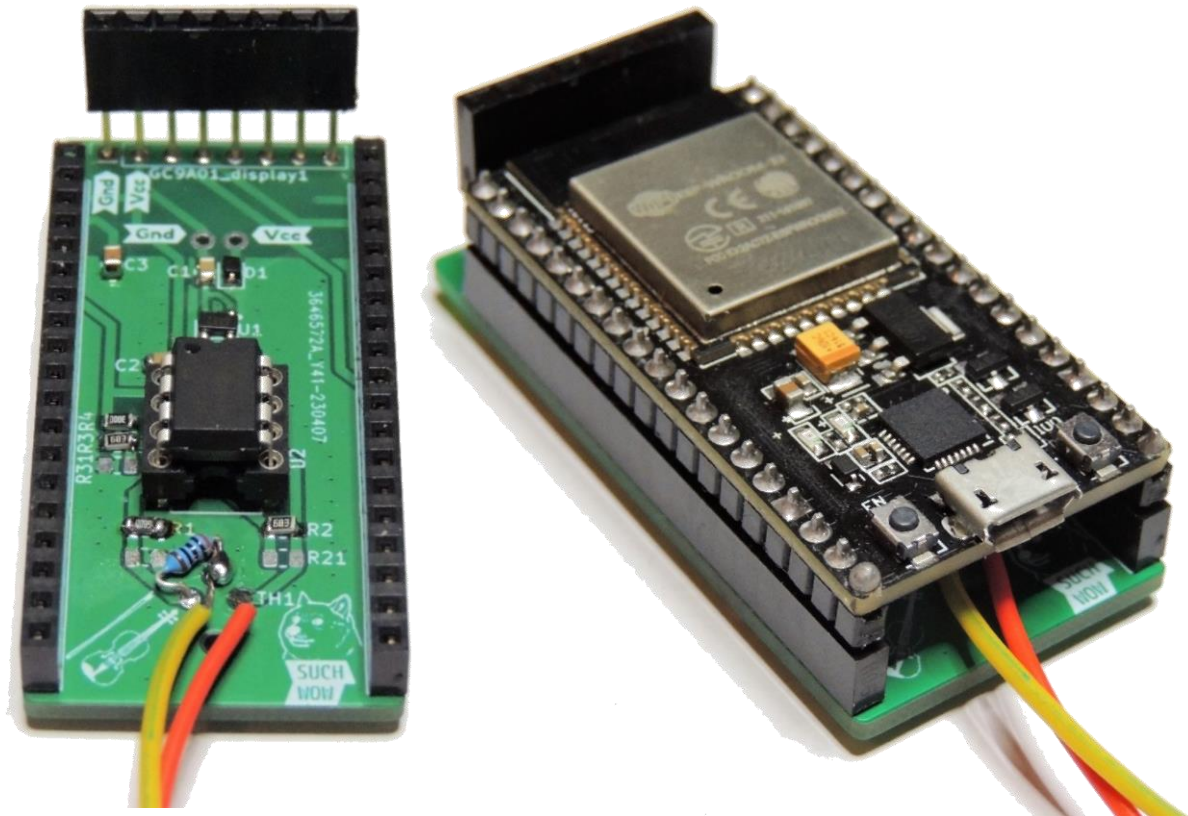
Obrázek 6.3 Osazená deska plošného spoje.
