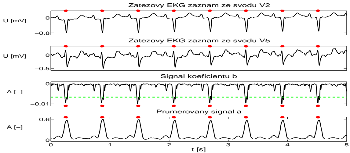
Obr. B.1: Ukázka výseku ze zátěžového záznamu ve svodu V2, V5 a signálech b , a_{avg} . F_{vz} = 5000Hz . Hlavní detekční svod: V2. Červené body představují nadetekované QRS komplexy. Zelená vodorovná čára v signálu b představuje práh detekce QRS.
