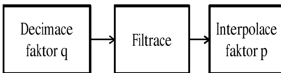
Obr. 3.2: Schéma způsobu filtrace signálu.
