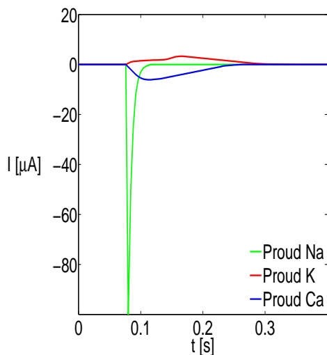
Obr. 2.1: Proudů jednotlivých iontů při depolarizaci.
