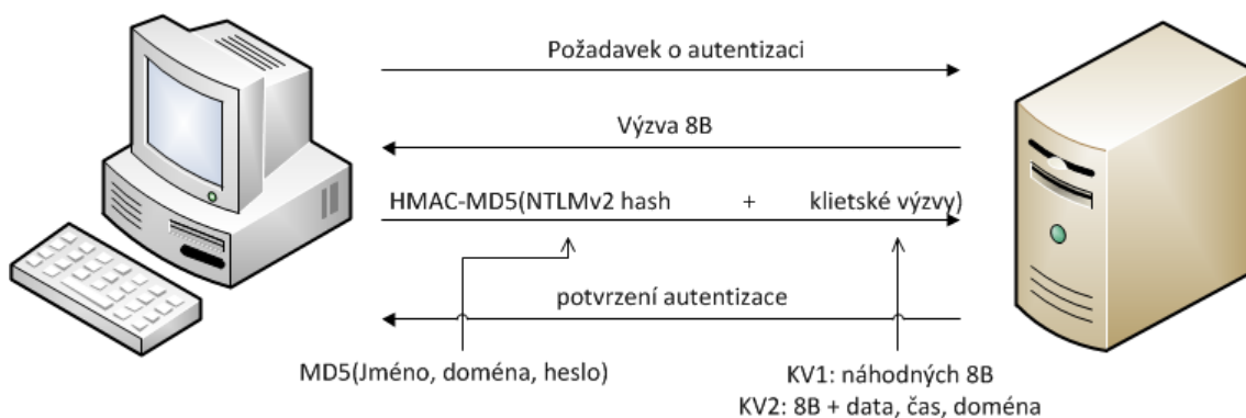
Obr. 2.4: NTLMv2 výzva-odpověď
