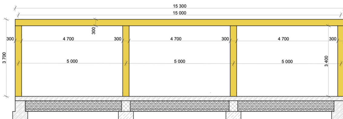
Obrázek 30 Geometrie vazby
