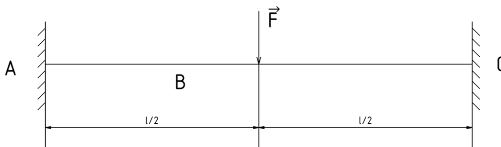
Obr. 37) Nahrazení lineárního vedení nosníkem [33]
