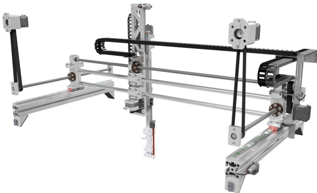
Obr. 34) Pohled na manipulátor zezadu
