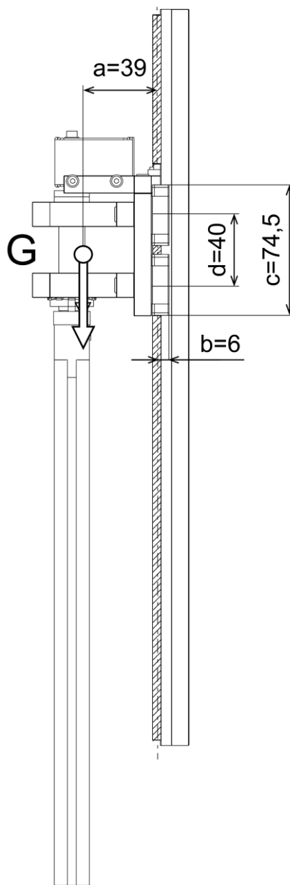
Obr. 39) Tíhová síla v těžišti smykadla
