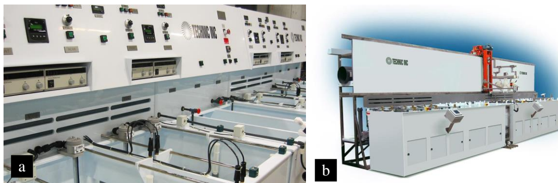
Obr. 6) a), b) Příklad poloautomatické linky pro elektrolytické leštění [42]
