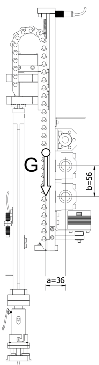
Obr. 38) Tíhová síla v těžišti sestavy
