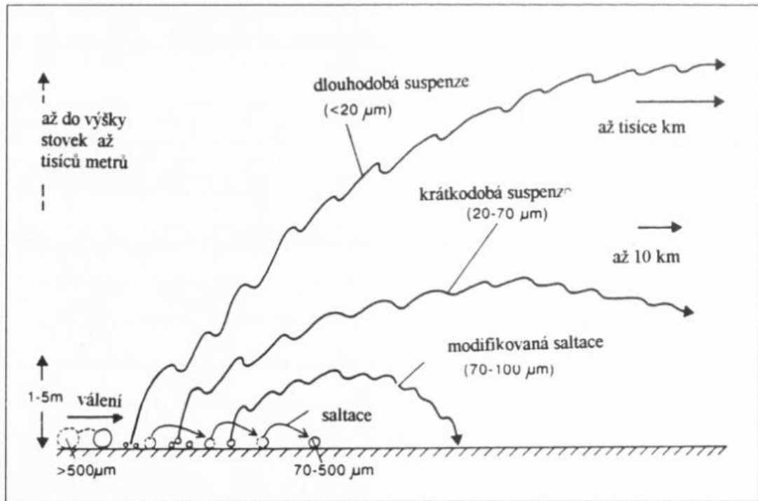
Obrázek 4 Různé způsoby eolického transportu siltu (jemného písku), písku, a šterku, během větrné bouře (rychlost větru od 10 do 20 cm/s). Podle Pye 1987 in Einselle 1992. (Kachlík, Chlupáč 1996)
