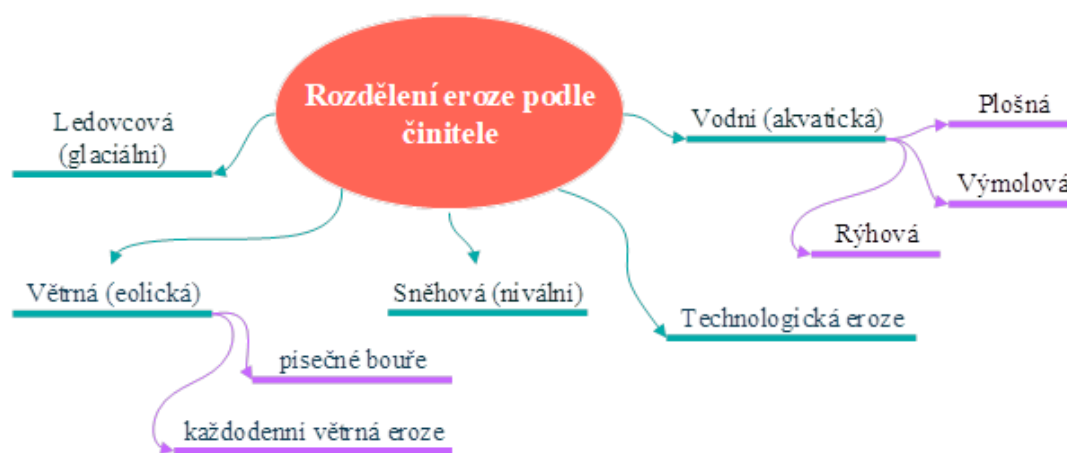
Obrázek 3 Rozdělení eroze podle činitele
