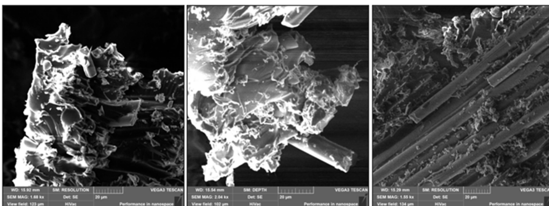
Obr. 28 Tříška nástroje HSS, SK, HSS+
