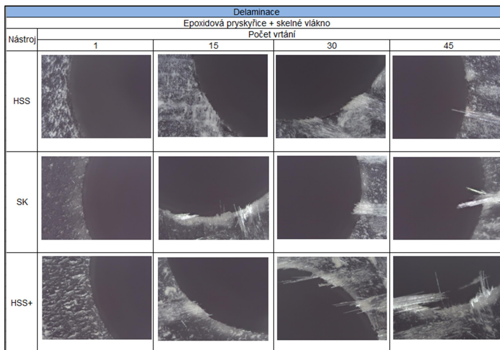
Obr. 24 Delaminace při vrtání do Vzorku A.
