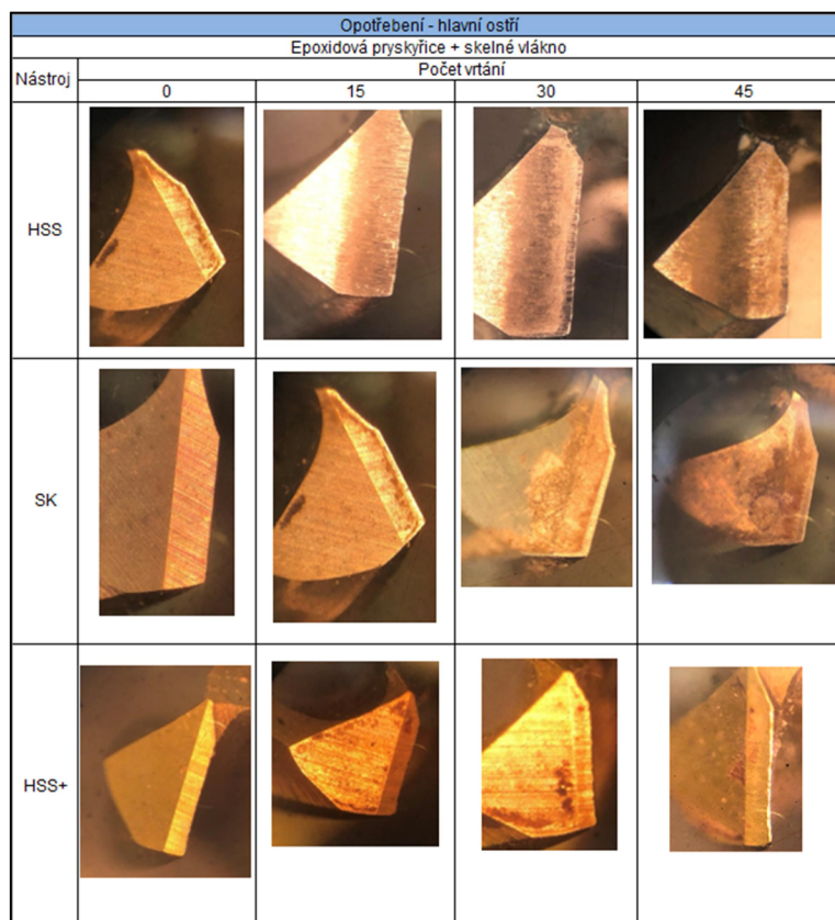
Obr. 20 Opotřebení hlavního ostří rezných nástrojů při vrtání do Vzorku A.
