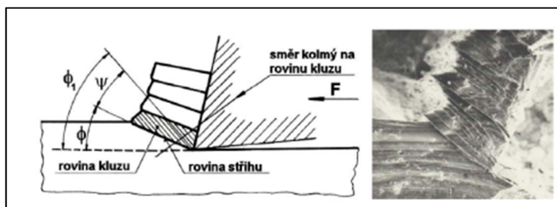
Obr. 8 Vznik třísky [9]
