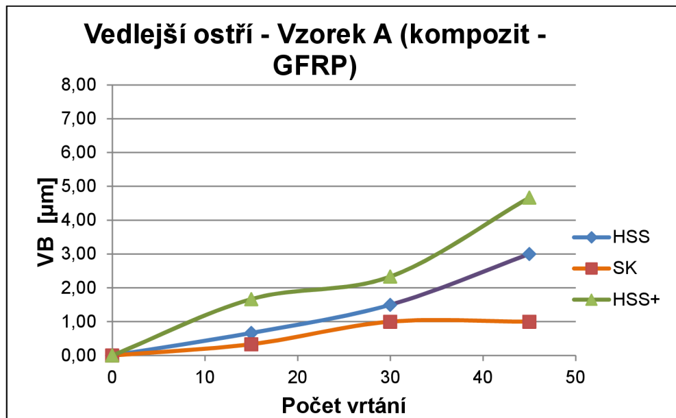
Graf 2 Naměřené hodnoty opotřebení na vedlejší ostří při vrtání do Vzorku A.
