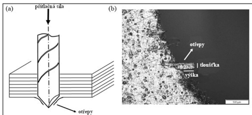
Obr. 6 (a) Tvorba otřepů při vrtání; (b) snímek otřepů z optického mikroskopu. [1]
