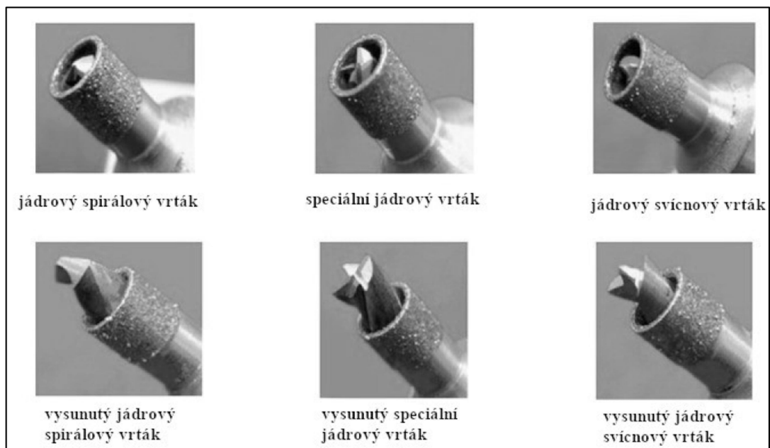
Obr. 3 Jádrové vrtáky [4]
