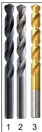
Obr. 14 Řezné nástroje
