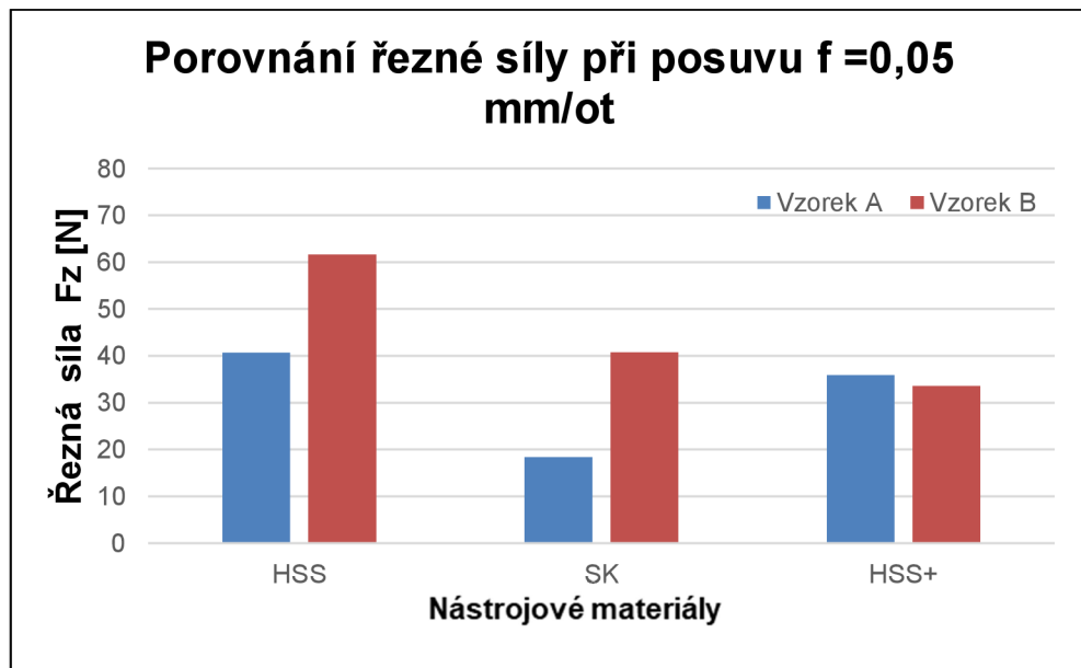
Graf 11 Porovnání řezné síly při posuvu f = 0,05 [mm/ot].
