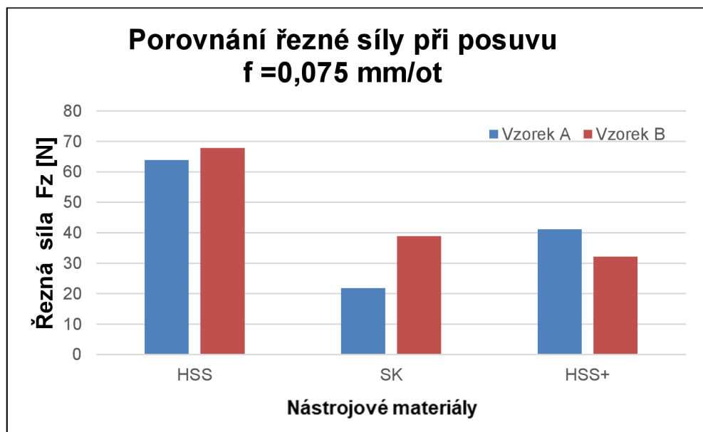
Graf 12 Porovnání řezné síly při posuvu f = 0,075 [mm/ot].
