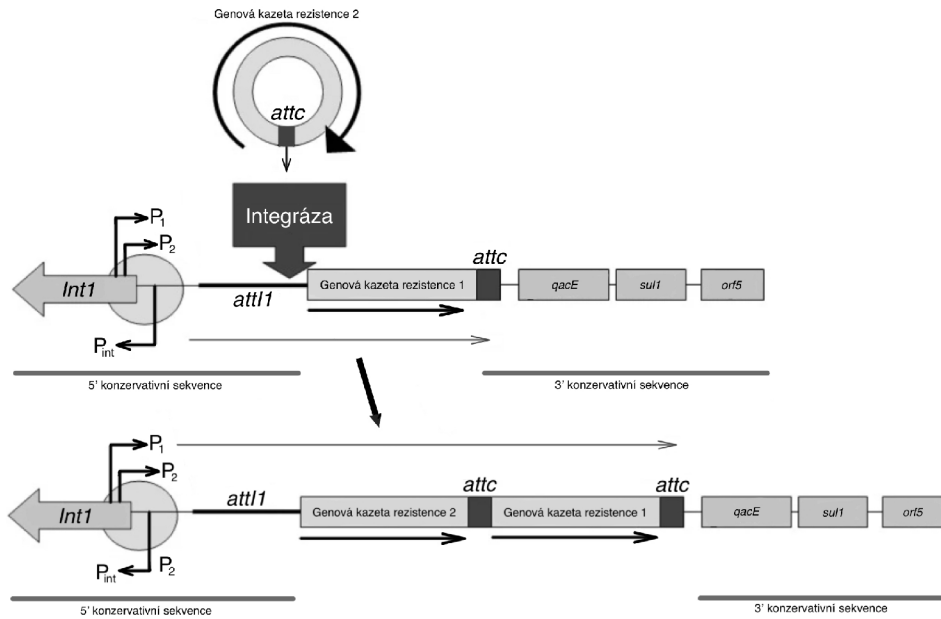
Obr. 1.5: Struktura integronu a integrace genových kazet[18]
