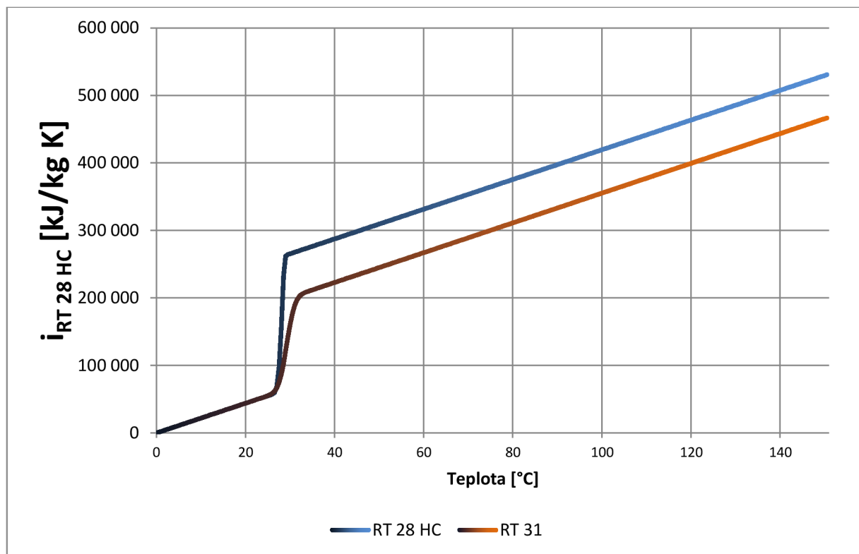
Graf 2: Entalpie RT parafinu od Rubitherm.
