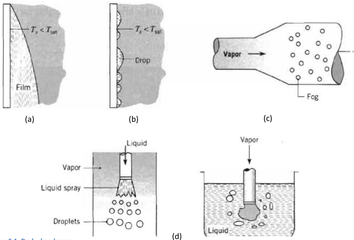
Obr. 5.1: Druhy kondenzace
