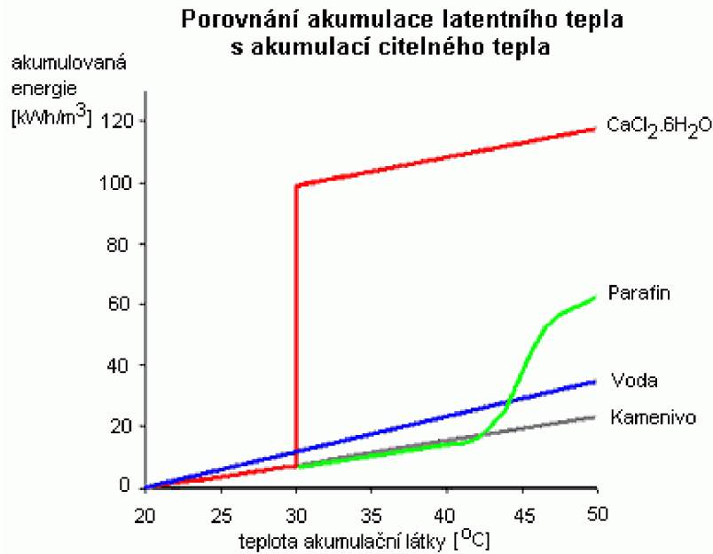
Obrázek 4.1: Graf porovnání materiálů s PCM.
